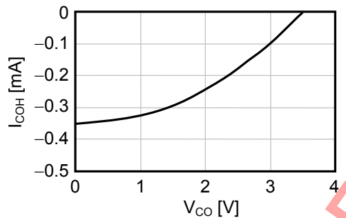
3.1 I_{COH}-V_{CO}
