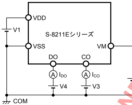
図7 測定回路3
