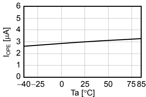
1.1 I_{OPE}-T_a
