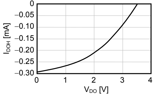
3.3 I_{DOH} - V_{DO}
