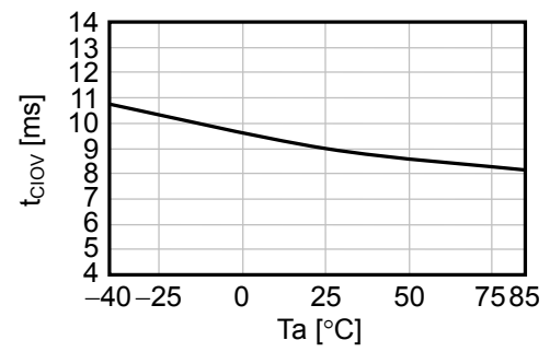
2.12 t_{CIOV} - T_a
