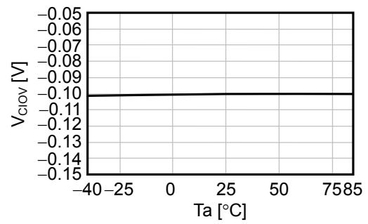
2.10 V_{CIOV} - T_a
