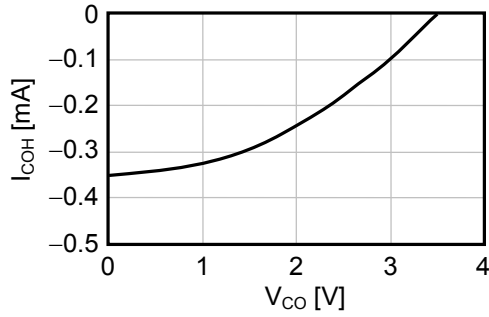
3.1 I_{COH} - V_{CO}
