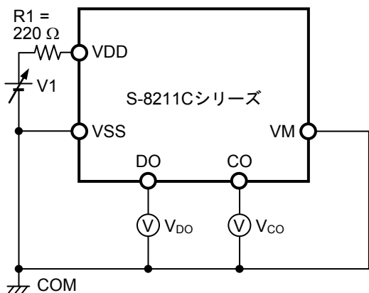
図5 測定回路1
