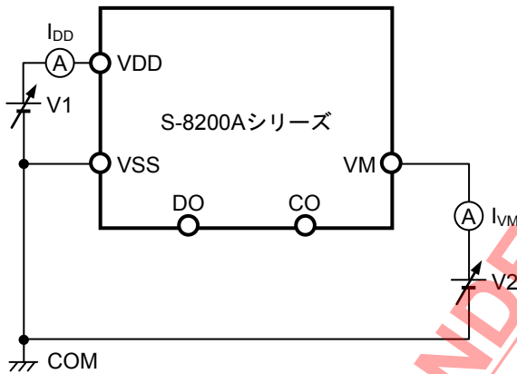
図7 測定回路3
