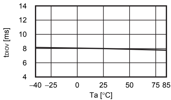
2. 9 t_{DIOV} - T_a
