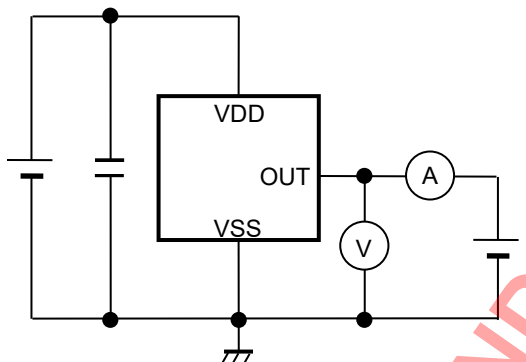
図7 測定回路3
