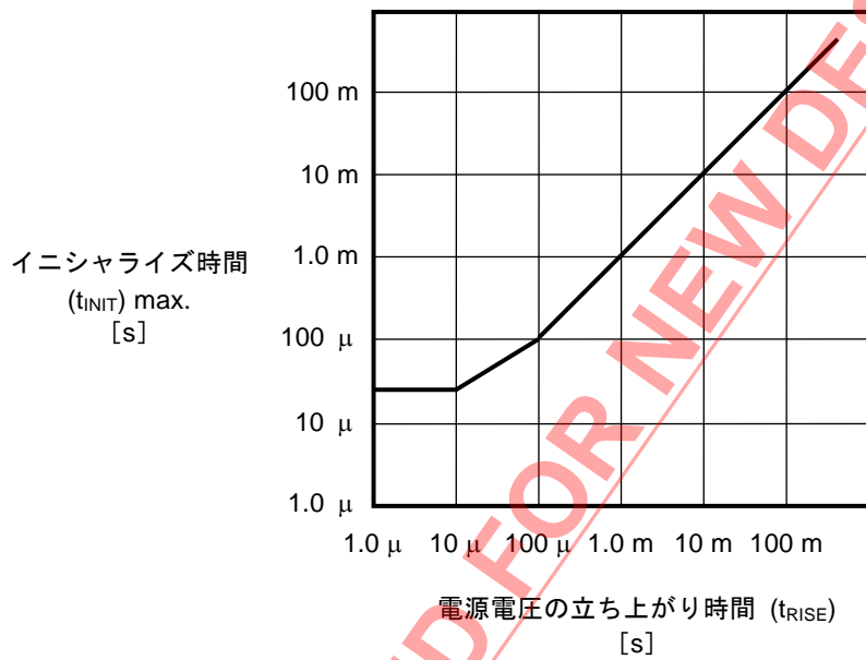
図28 S-24C16Cのイニシャライズ時間
