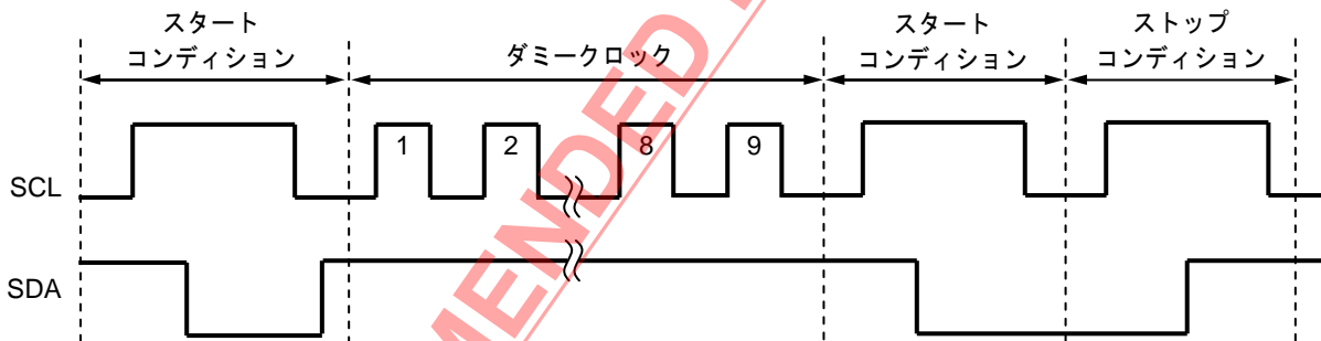
図25 S-24C16Cのリセット方法
