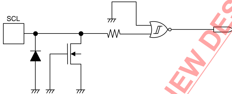
図22 SCL端子
