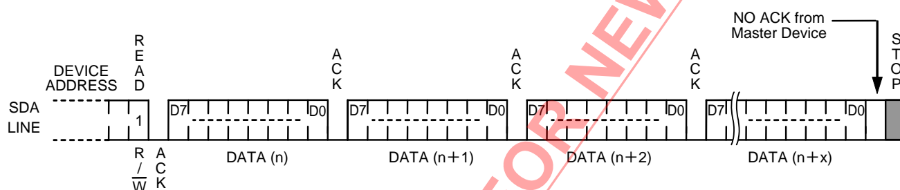
図20 シーケンシャルリード
