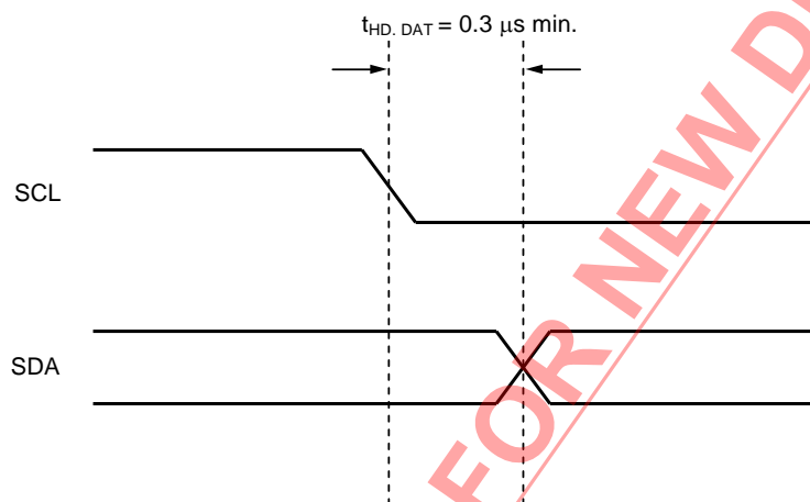
図29 S-24C16Cのデータホールド時間
