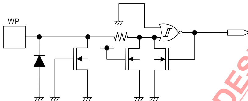
図24 WP端子
