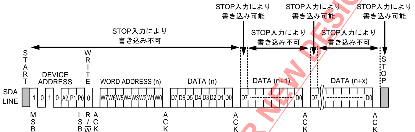
図32 書き込み中のストップコンディション入力による書き込み実行
