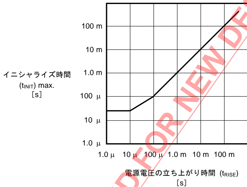
図29 S-24C08Cのイニシャライズ時間
