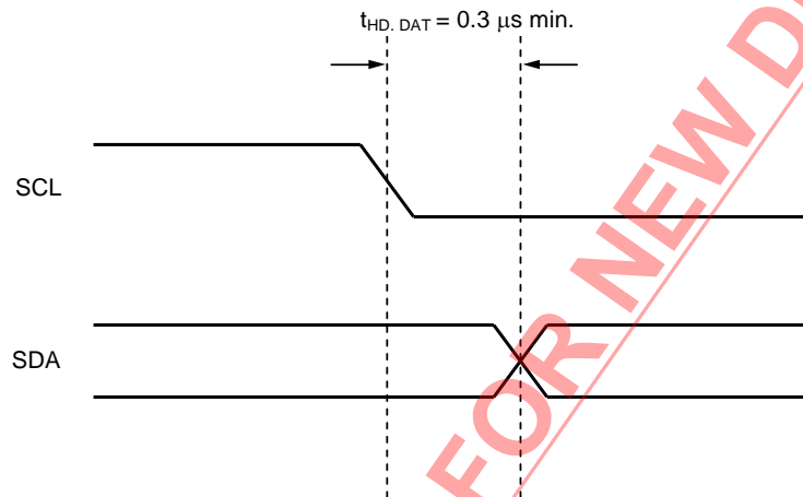
図30 S-24C08Cのデータホールド時間
