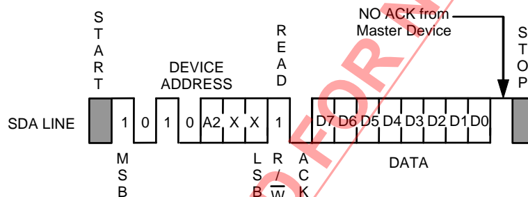
図18 カレントアドレスリード
