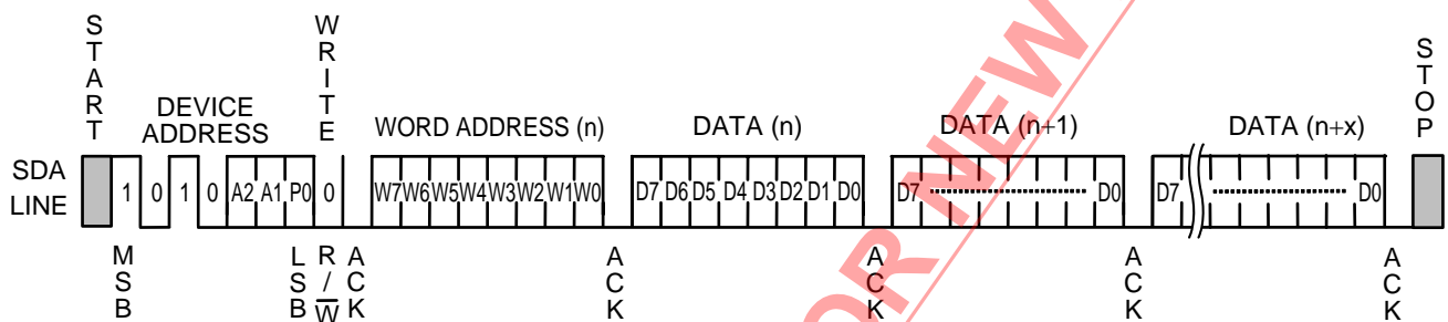
図15 ページライト
