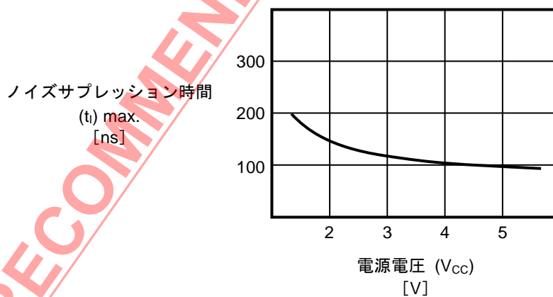
図 31 SDA 端子と SCL 端子ノイズサプレッション時間
