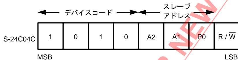
図13 デバイスアドレス
