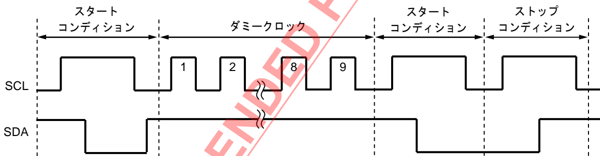
図 26 S-24C04C のリセット方法
