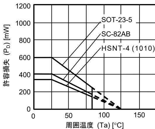
図8 パッケージ許容損失 (基板実装時)
