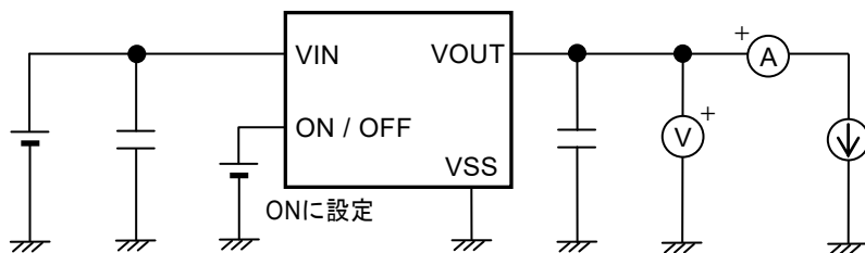
図10 測定回路1
