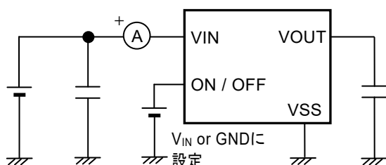
図11 測定回路2
