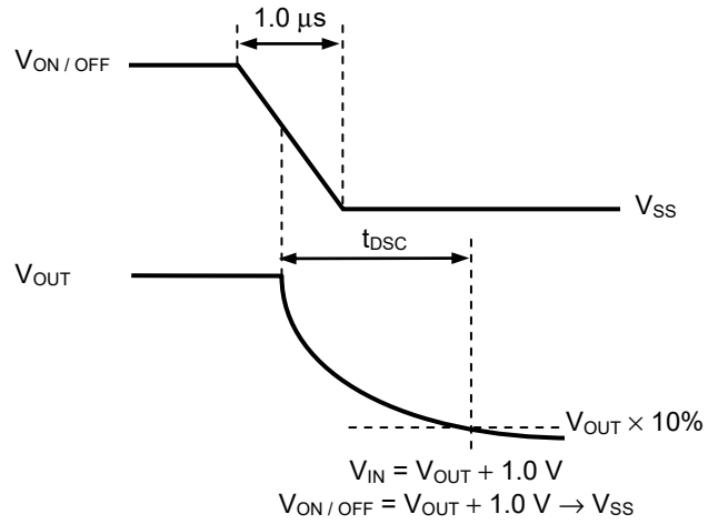
図27 放電時間の測定条件
