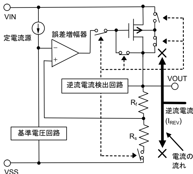
図23 逆流電流防止モード
