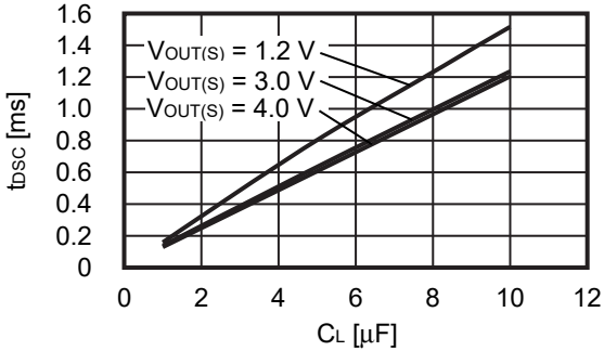
図26 S-13R1シリーズA/Bタイプ (放電シャント機能あり)
