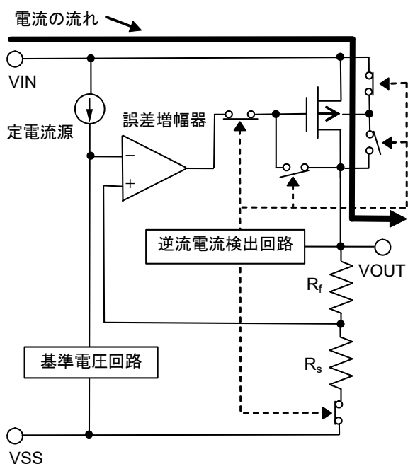
図22 通常動作モード
