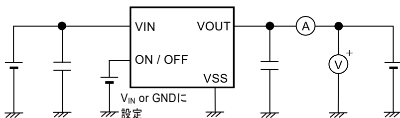
図12 測定回路3
