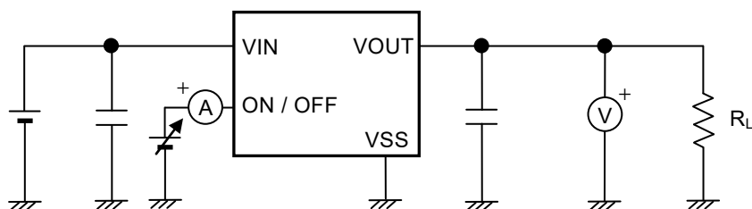
図13 測定回路4
