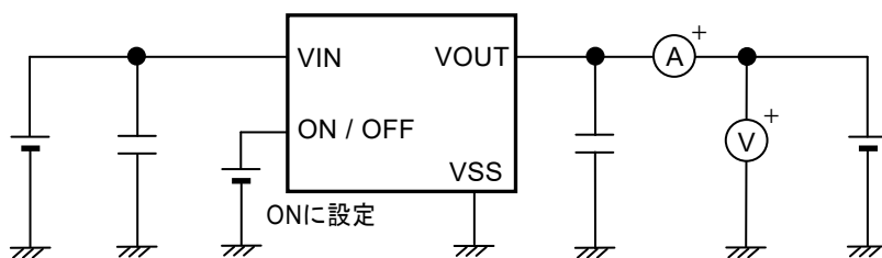
図15 測定回路6
