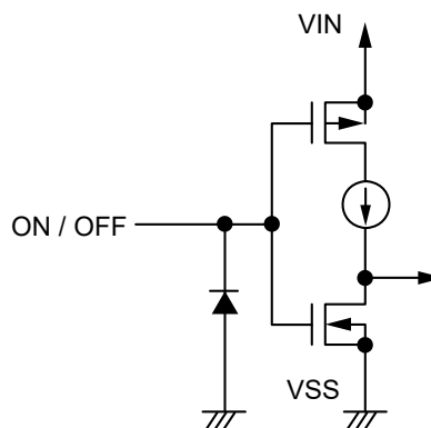
図20 S-13R1シリーズB / Dタイプ
