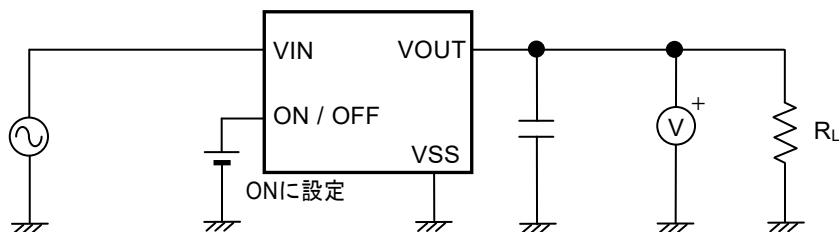
図14 測定回路5
