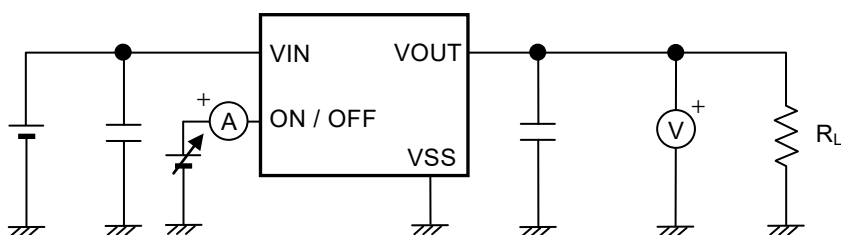
図11 測定回路4
