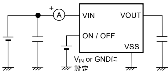
図9 測定回路2
