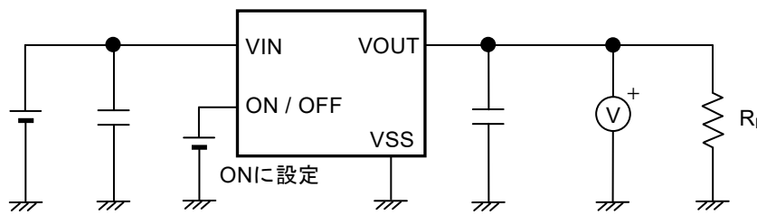
図13 測定回路6
