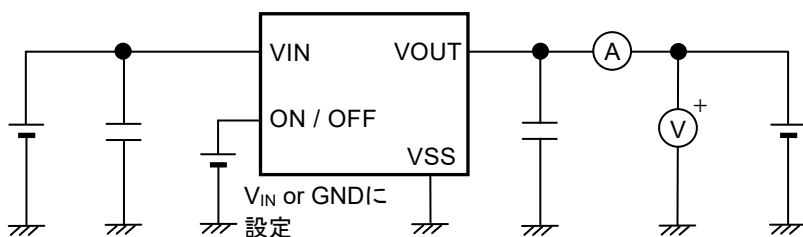
図10 測定回路3
