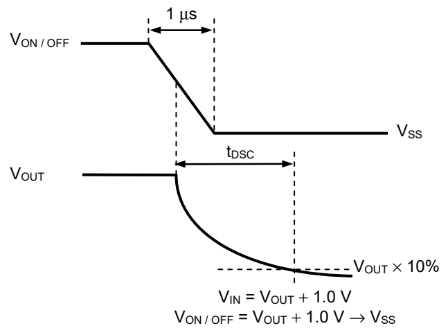
図21 放電時間の測定条件
