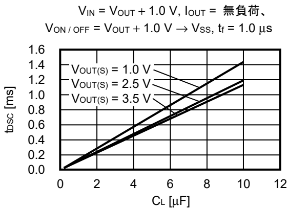
図20 S-1324シリーズA/Bタイプ (放電シャント機能あり)
