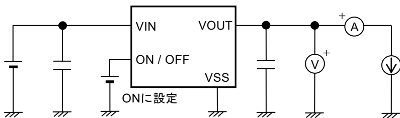
図8 測定回路1
