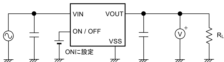
図12 測定回路5
