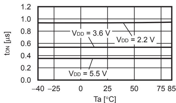
2.6 オン時間 (t ON ) - 温度 (Ta)
