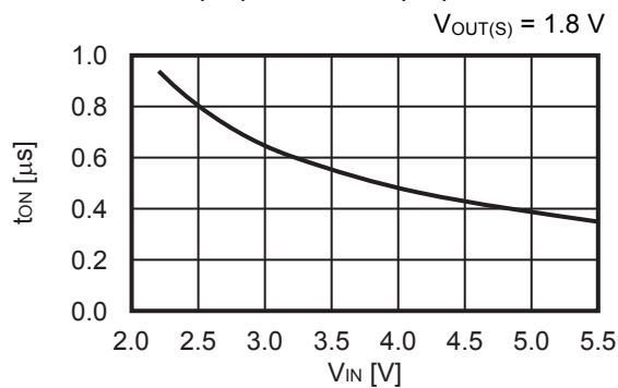
1.6 オン時間 ( t_{ON} ) – 入力電圧 ( V_{IN} )
