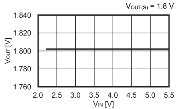
1.4 出力電圧 ( V_{OUT} ) – 入力電圧 ( V_{IN} )
