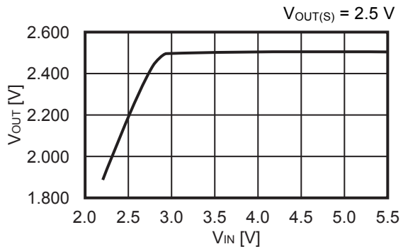
1.5 出力電圧 ( V_{OUT} ) – 入力電圧 ( V_{IN} )
