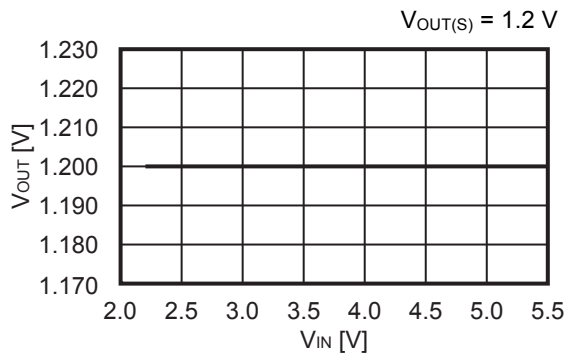
1.3 出力電圧 ( V_{OUT} ) – 入力電圧 ( V_{IN} )
