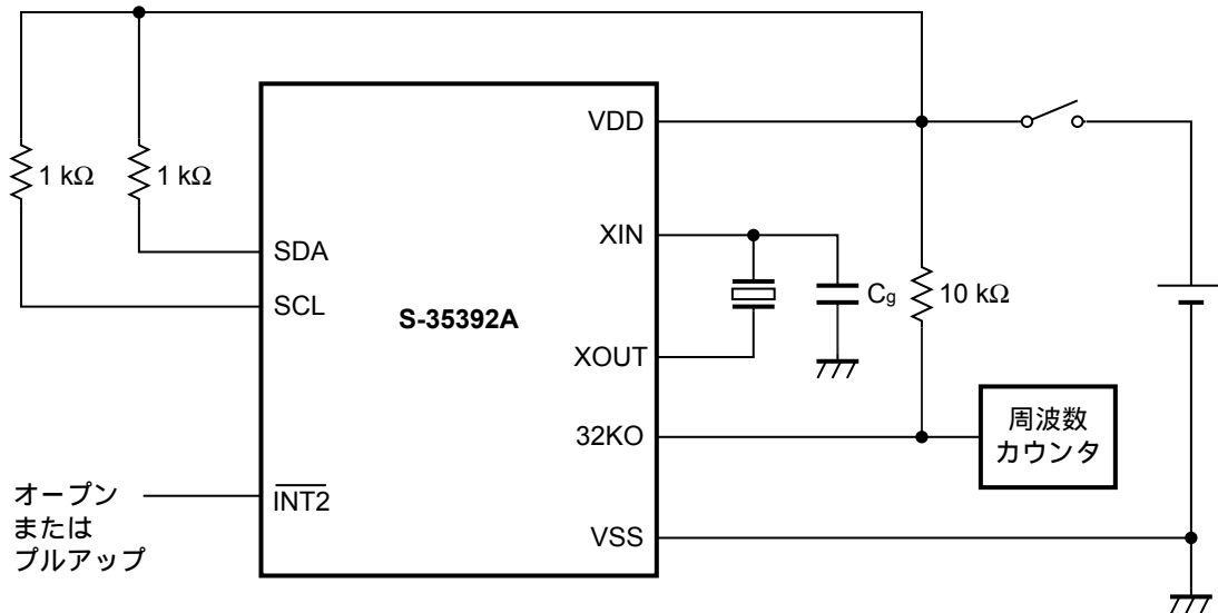
図48 発振周波数の測定回路構成
