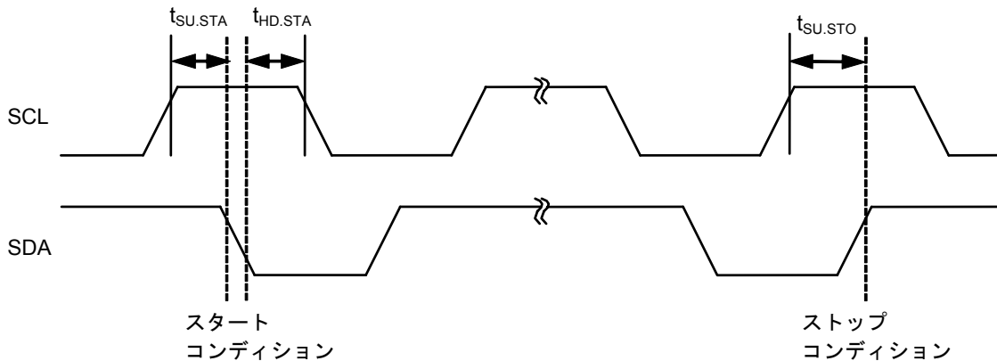
図29 スタート / ストップコンディション
