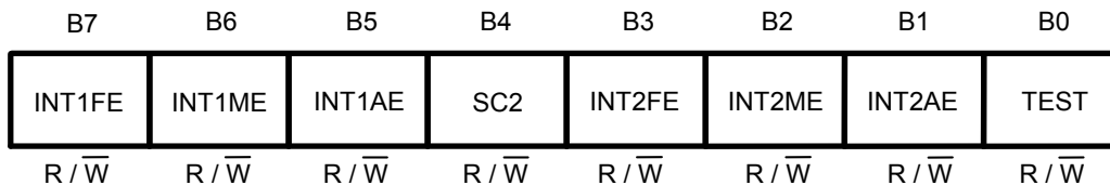
図11 ステータスレジスタ2
