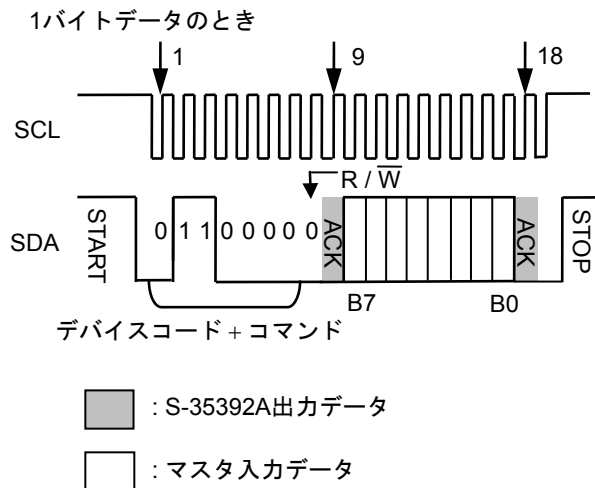
図33 データ書き込み例1 (1バイトデータレジスタ)
