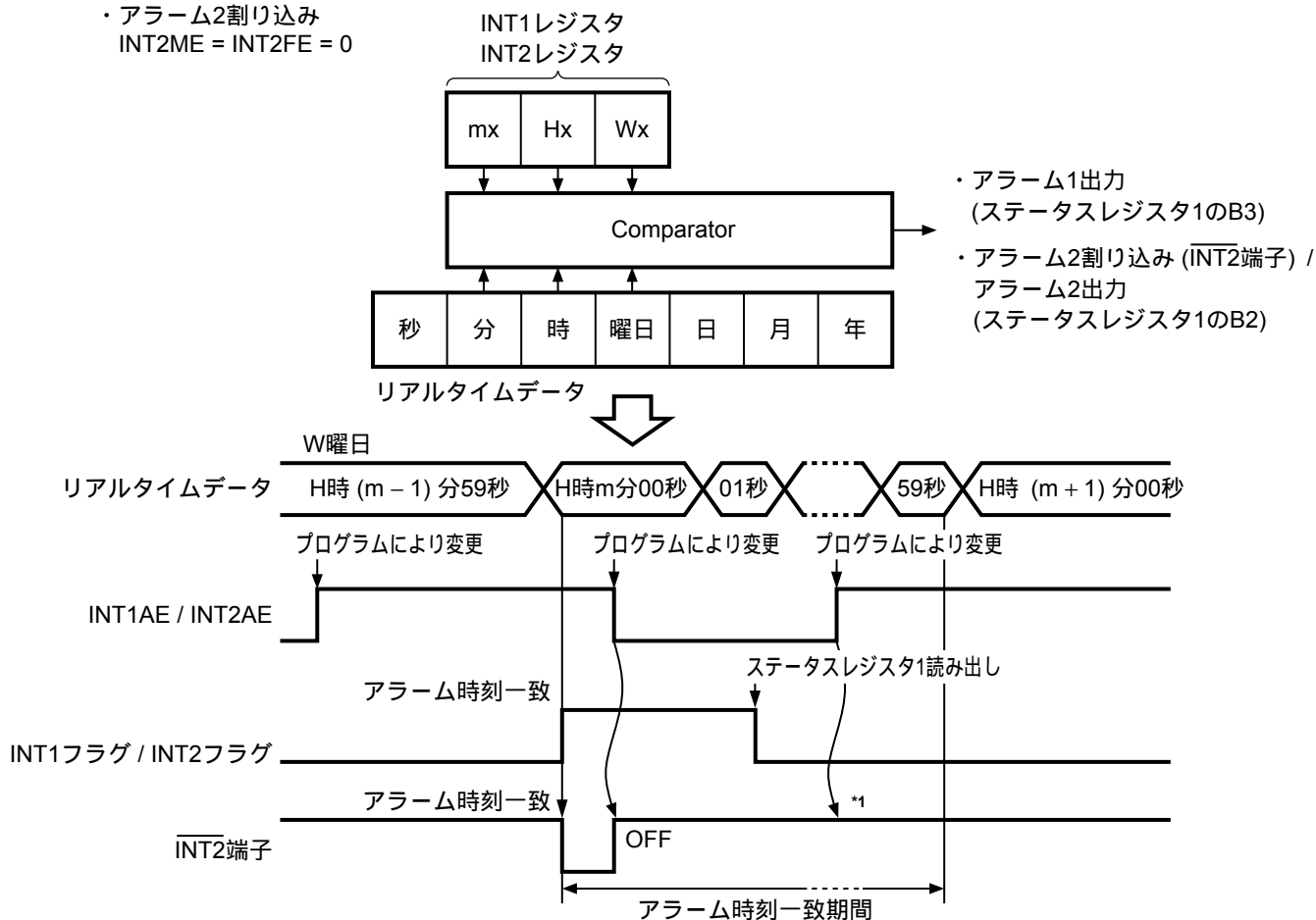
図23 アラーム割り込み出力タイミング
