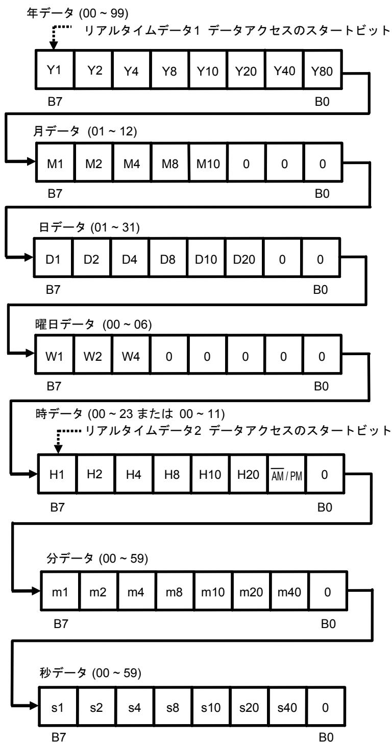
図9 リアルタイムデータレジスタ エイブリック株式会社
