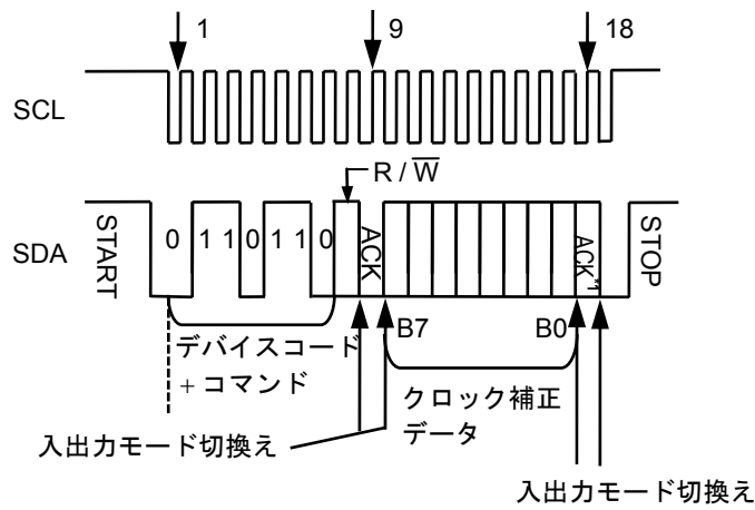
図40 クロック補正レジスタアクセス
