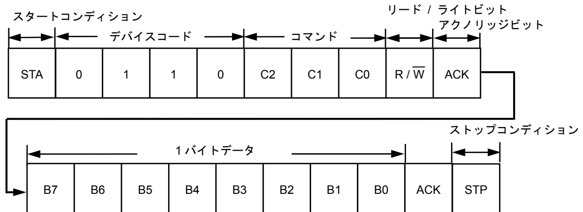
図8 通信データ
