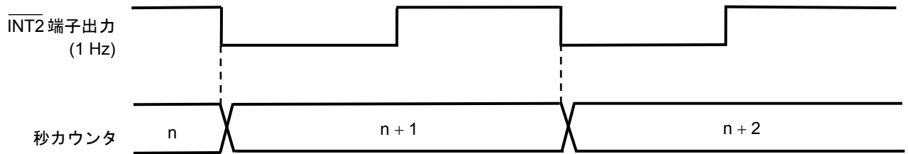
図16 1 Hzのクロック出力と秒カウンタ
