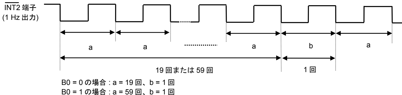
図28 クロック補正確認方法
