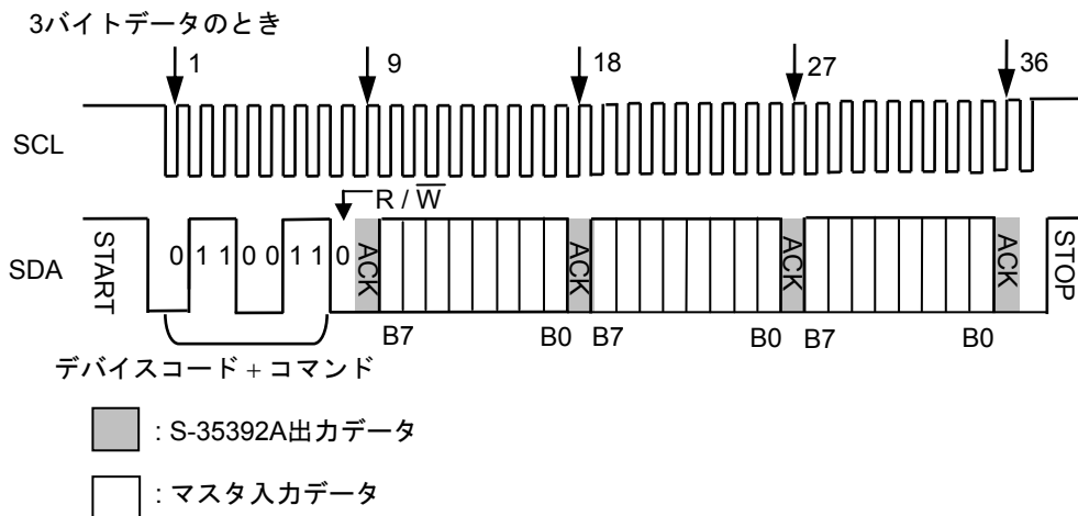
図34 データ書き込み例2 (3バイトデータレジスタ)
