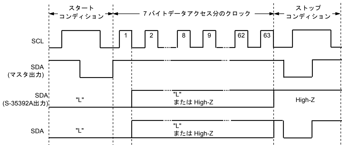
図42 リセット処理方法
