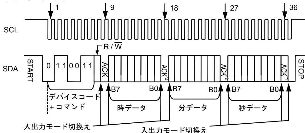
図35 リアルタイムデータ1アクセス
