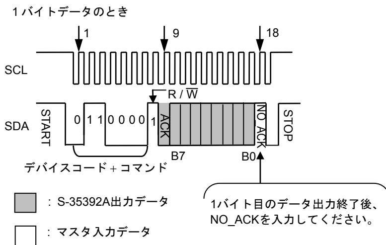
図31 データ読み出し例1 (1バイトデータレジスタ)
