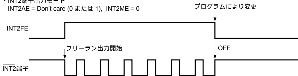
図25 周波数設定出力タイミング
