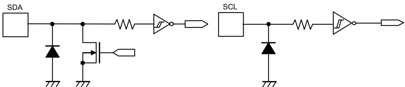
図3 SDA端子
