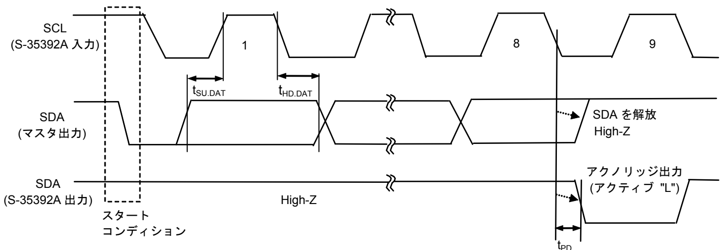
図30 アクノリッジ出力タイミング
