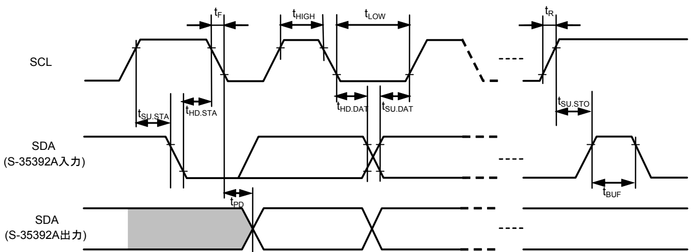
図7 バスタイミング
