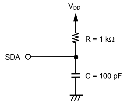
図6 出力負荷回路
