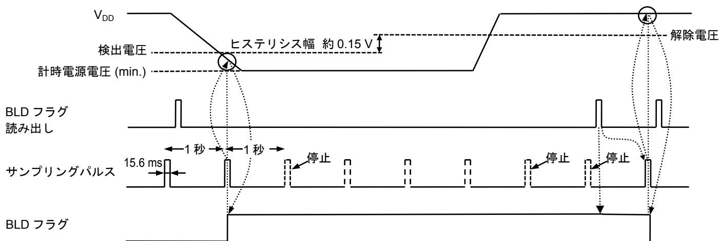
図21 低電源電圧検出回路タイミング
