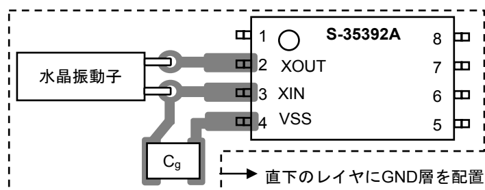
図47 接続図2
