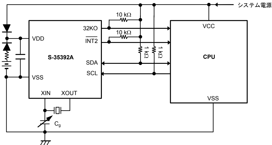
図45 応用回路2
