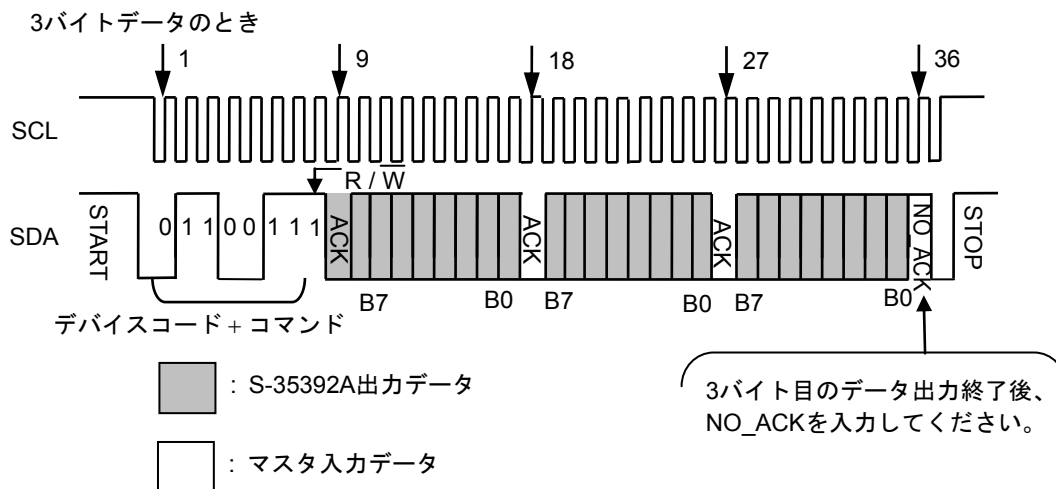
図32 データ読み出し例2 (3バイトデータレジスタ)
