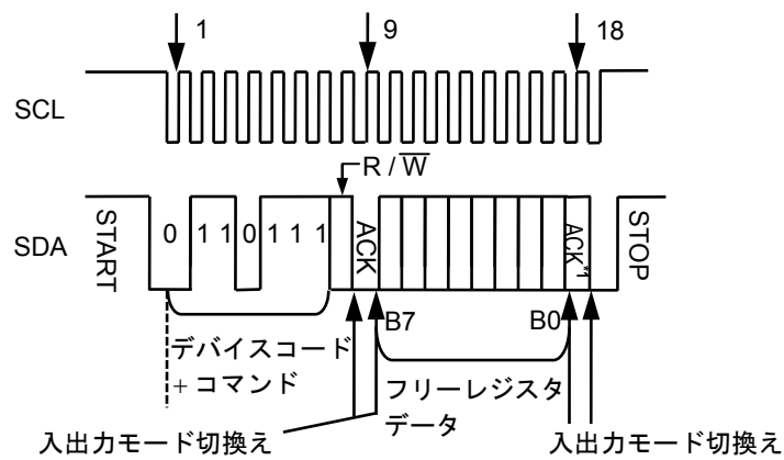
図41 フリーレジスタアクセス
