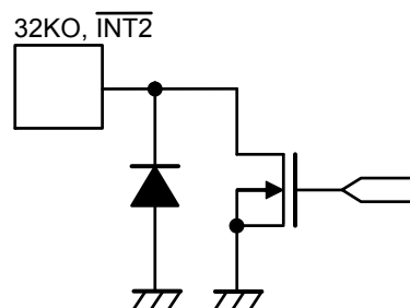
図5 32KO端子、INT2端子
