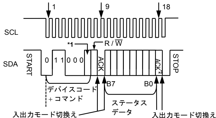
図36 リアルタイムデータ2アクセス
