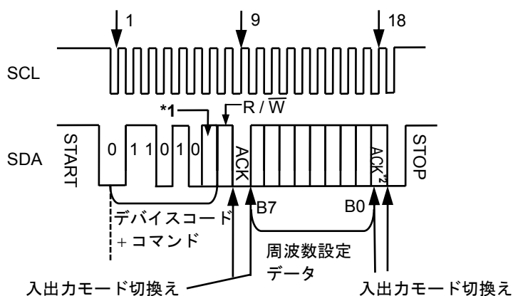
図38 INT1レジスタアクセス、INT2レジスタアクセス
