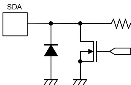
図4 SDA端子
