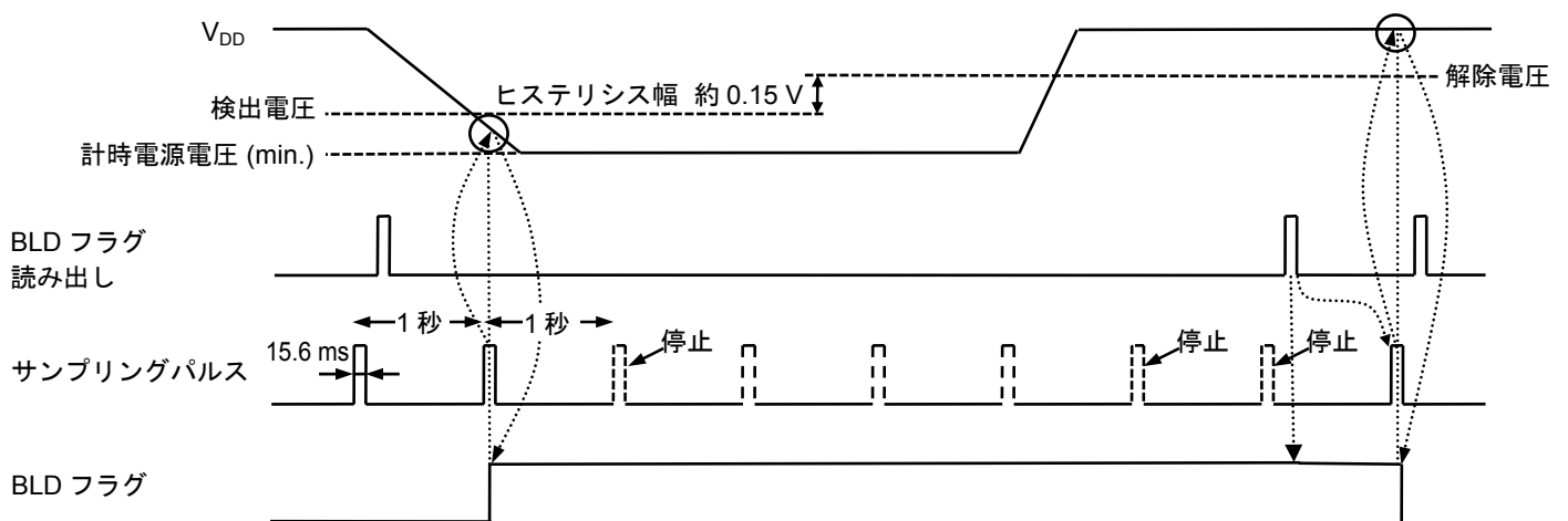
図22 低電源電圧検出回路タイミング
