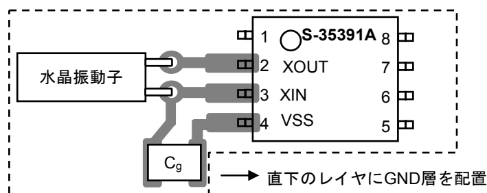
図50 接続図2
