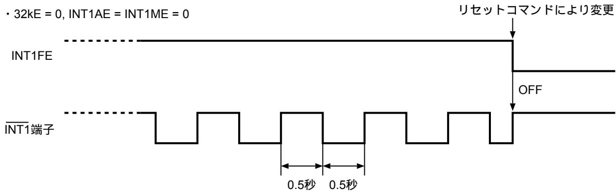
図30 パワーオン検出回路動作時の \overline{\text{INT1}} 端子出力タイミング
