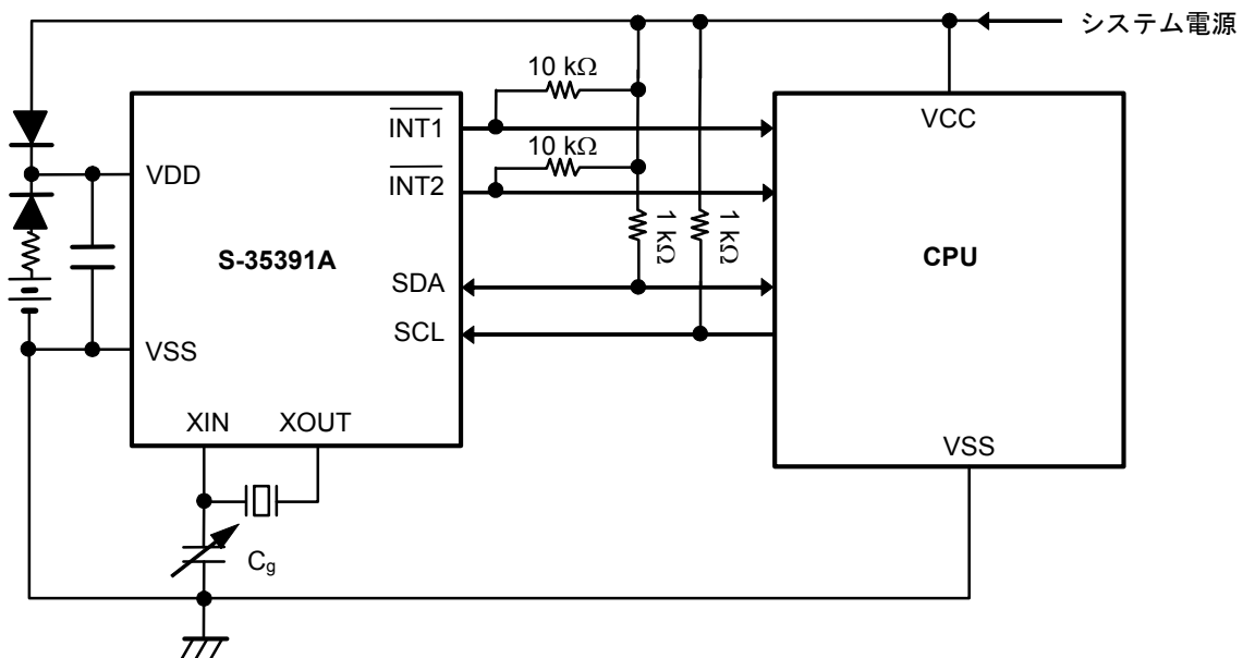
図48 応用回路2
