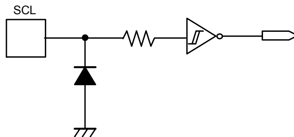
図5 SCL端子
