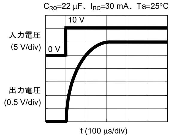
図12 電源投入のリングング波形（VRO端子）
