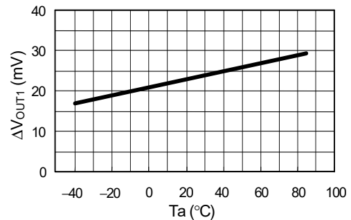
1.12 負荷安定度 ( V_{OUT} ) 温度特性
