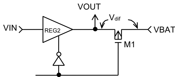
図8 V_{dif} の定義
