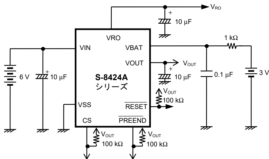
図21 標準回路
