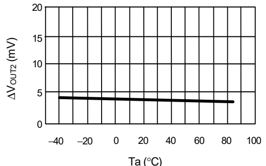
1.12 負荷安定度 ( V_{OUT} ) 温度特性
