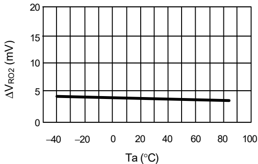
1.11 負荷安定度 ( V_{RO} ) 温度特性
