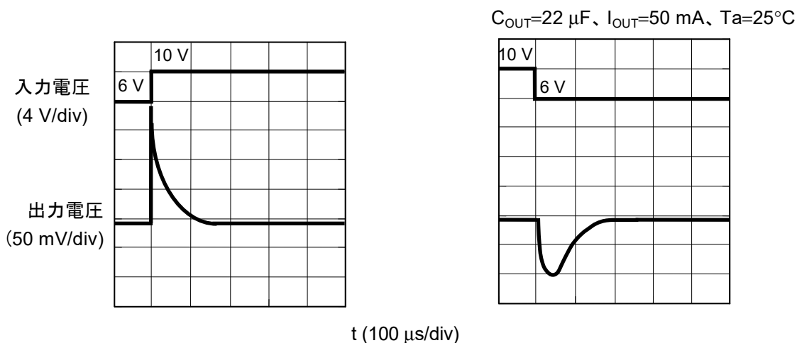
図15 電源変動のリングング波形 (VOUT端子)
