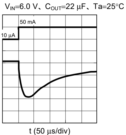
図19 負荷変動によるリングング波形 (VOUT端子)
