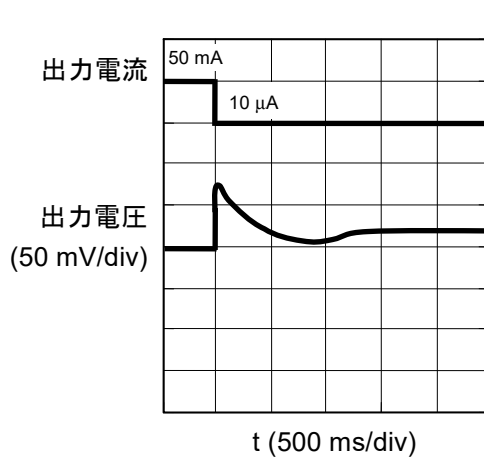
図19 負荷変動によるリングング波形 (VOUT端子)
