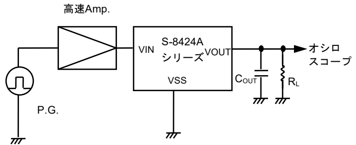
図10 測定回路
