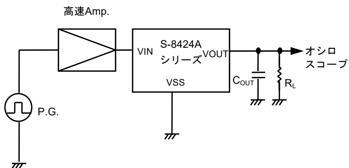
図14 測定回路
