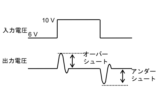
図13 電源変動：6 V↔10 Vの矩形波の場合
