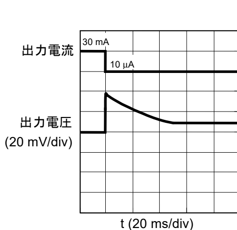
図20 負荷変動によるリングング波形 (VRO端子)
