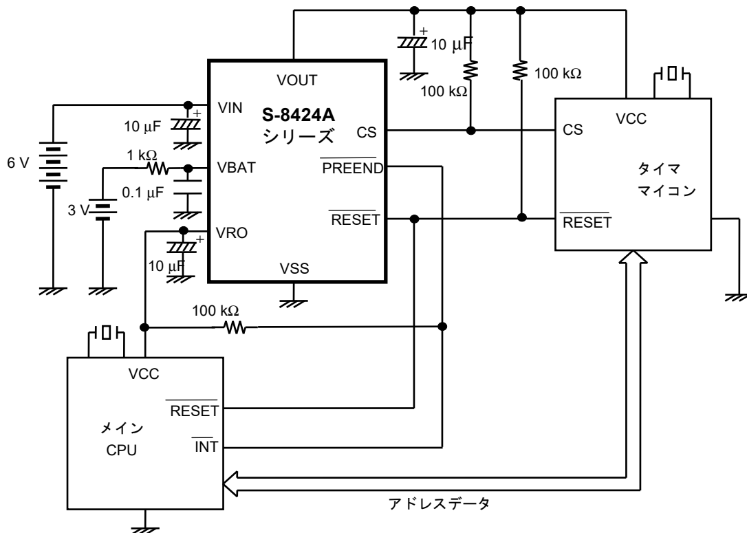
図22 応用回路1
