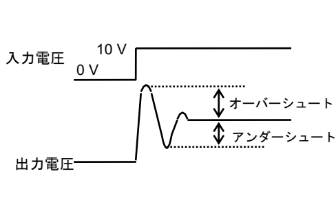
図9 電源投入：0 V→10 Vの矩形波の場合
