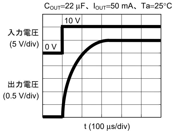
図11 電源投入のリングング波形（VOUT端子）
