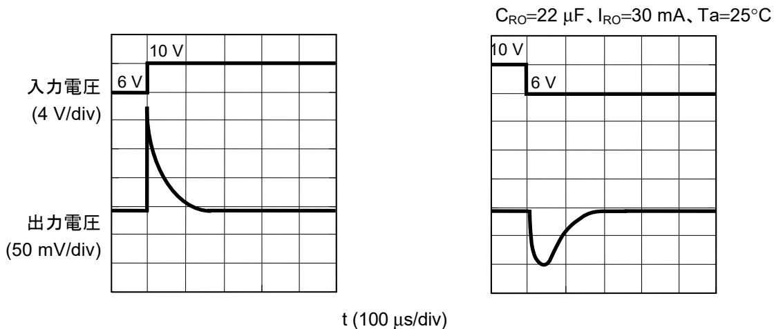
図16 電源変動のリングング波形 (VRO端子)
