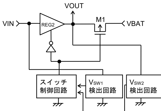
図7 スイッチ部
