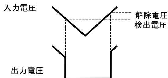
図6 電圧検出器の検出と解除電圧の定義
