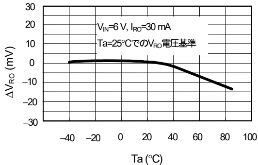
1.9 入力安定度 ( V_{RO} ) 温度特性
