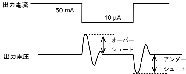
図17 出力電流による出力電圧の変動
