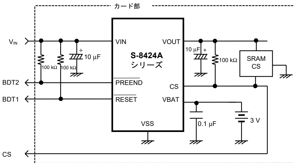
図24 応用回路3
