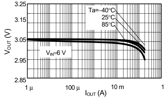
1.8 出力電圧 ( V_{OUT} ) 温度特性
