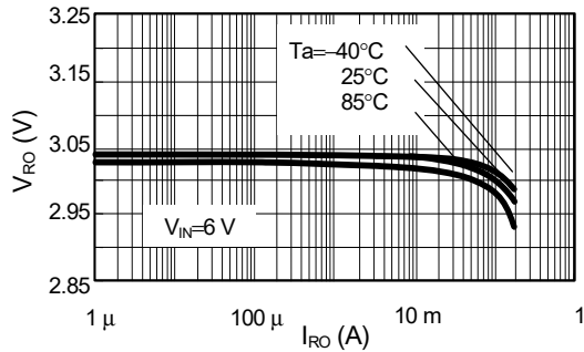
1.7 出力電圧 ( V_{RO} ) 温度特性
