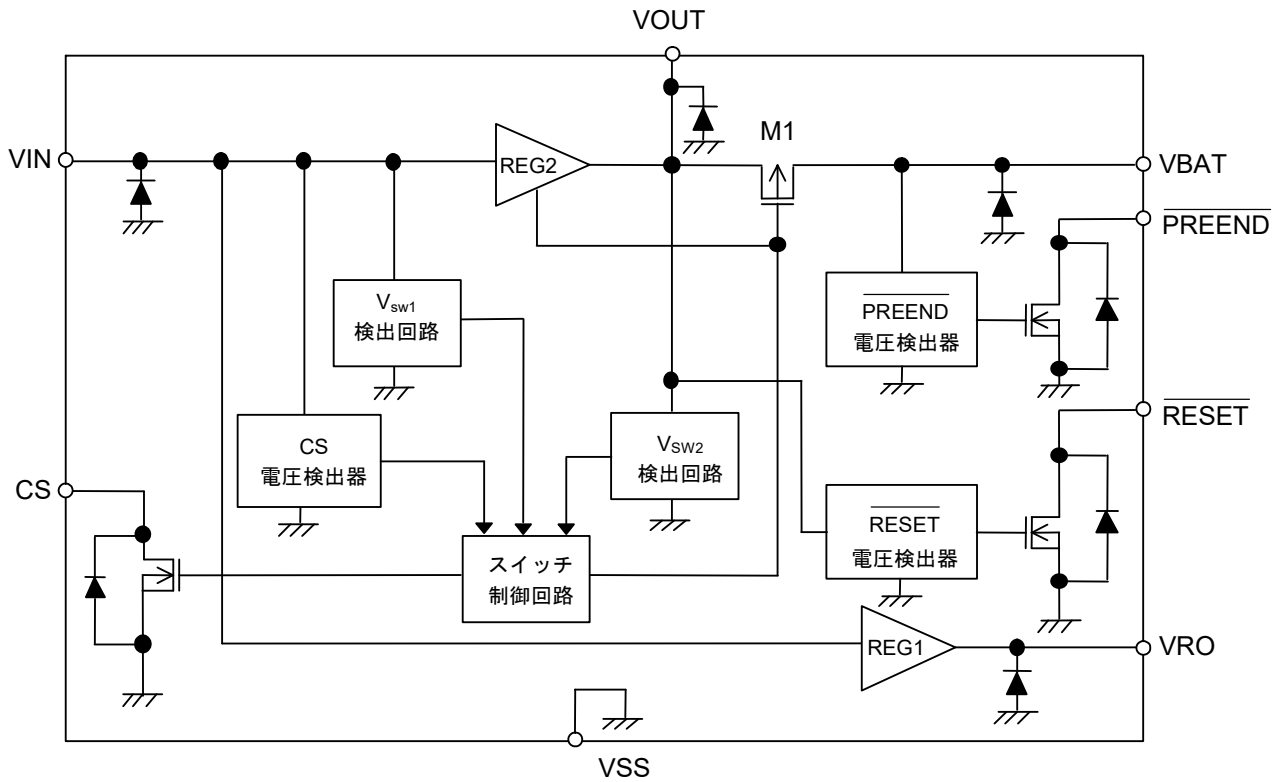
図1 ブロック図
