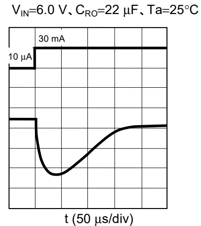
図20 負荷変動によるリングング波形 (VRO端子)
