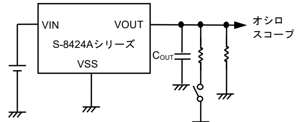
図18 測定回路
