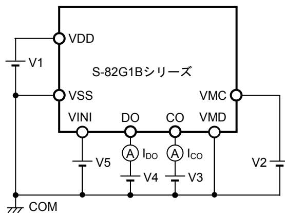
図6 測定回路4
