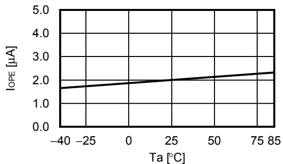
1.1 I_{OPE} - T_a
