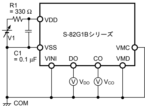
図3 測定回路1
