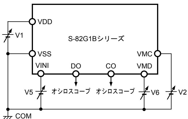
図7 測定回路5
