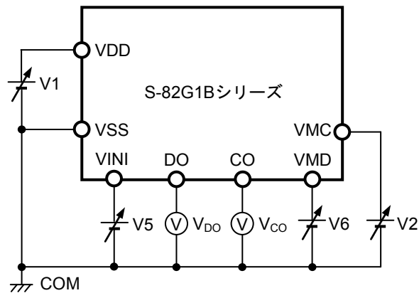
図4 測定回路2
