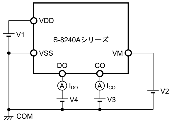
図9 測定回路4
