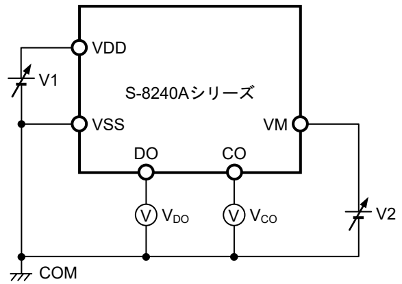
図7 測定回路2
