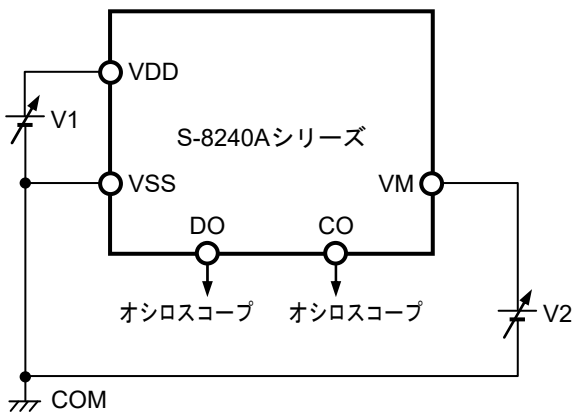
図10 測定回路5
