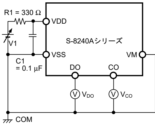
図6 測定回路1
