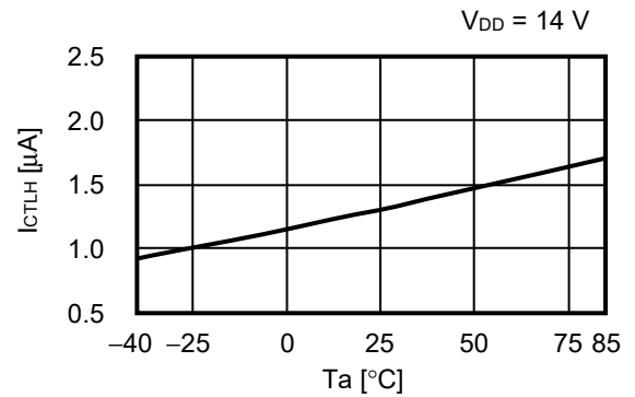
4.2 I_{CTLH} - T_a
