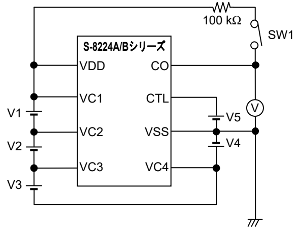
図6 測定回路2
