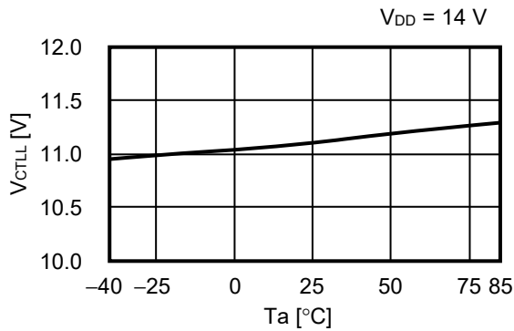
4.1 V_{CTL} - T_a
