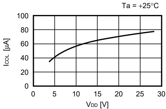
5.3 I_{COL} - V_{DD}
