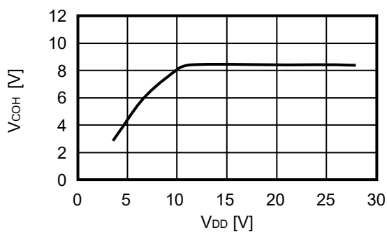
6.1 V_{COH} - V_{DD}
