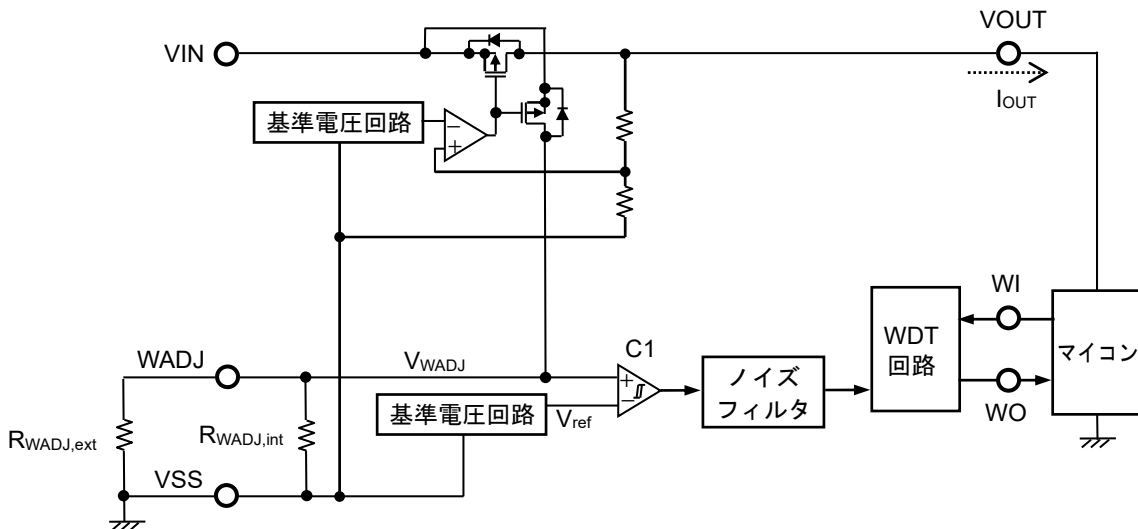
図49 出力電流検出回路の動作説明図
