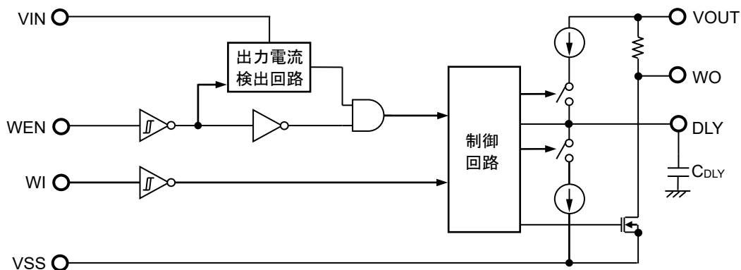
図43 ウォッチドッグタイマ部の動作説明図
