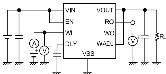
図33 測定回路11
