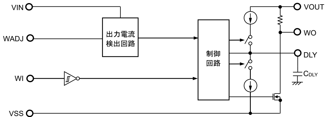
図48 ウォッチドッグタイマ部の動作説明図
