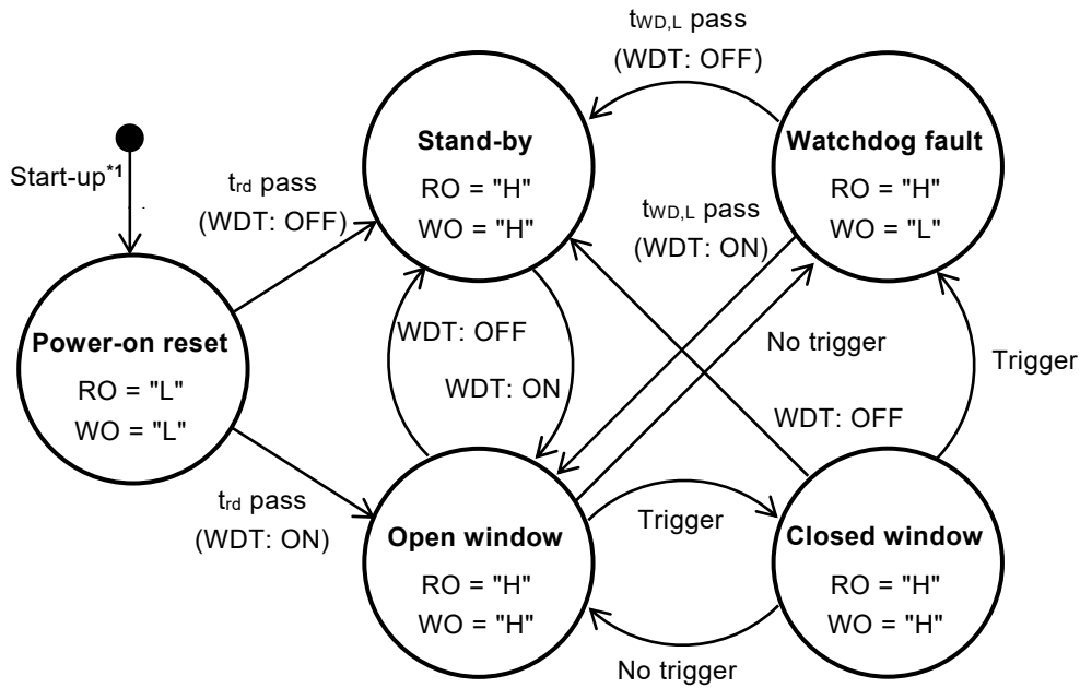
図47 ウォッチドッグタイマ部の状態遷移図
