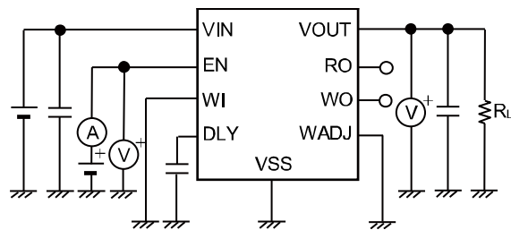
図26 測定回路4
