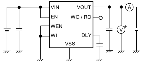
図14 測定回路2
