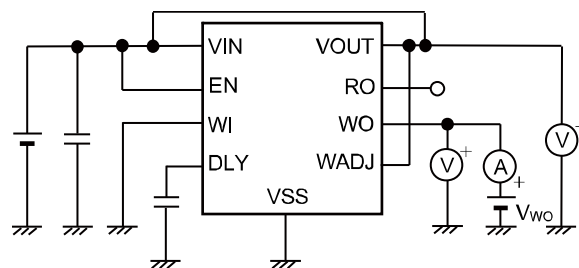
図34 測定回路12
