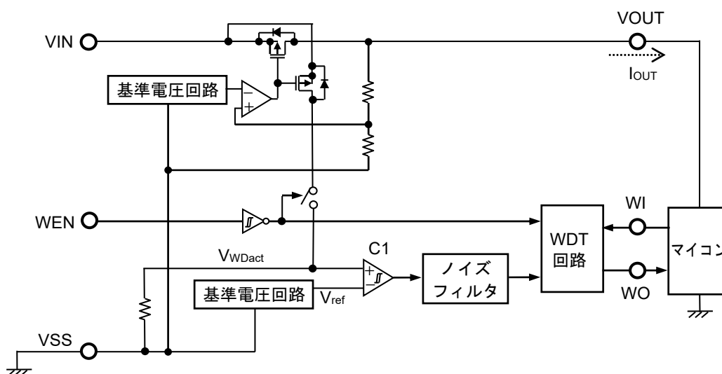
図44 出力電流検出回路の動作説明図
