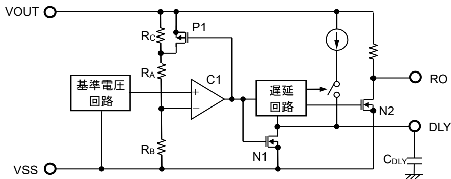
図39 ディテクタ部の動作説明図
