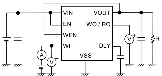
図19 測定回路7
