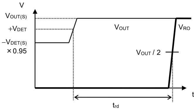
図7 解除遅延時間
