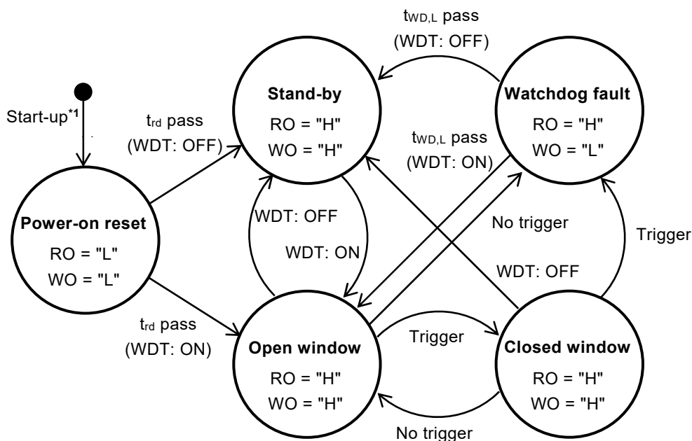
図42 ウォッチドッグタイマ部の状態遷移図
