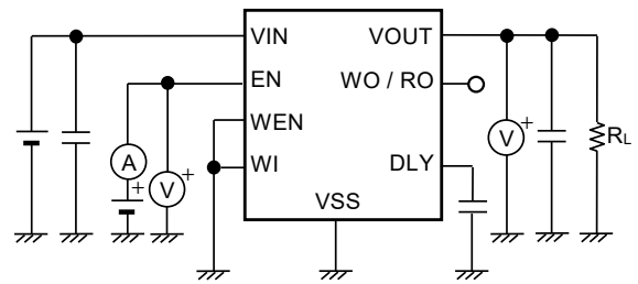
図16 測定回路4
