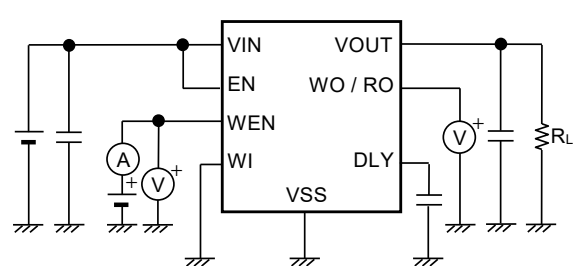
図20 測定回路8
