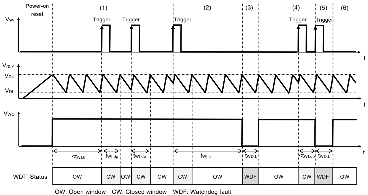
図46 ウォッチドッグタイマ部のタイミングチャート
