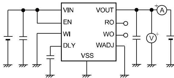
図24 測定回路2
