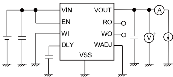
図23 測定回路1
