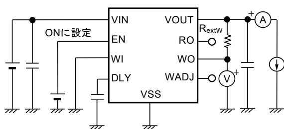
図29 測定回路7
