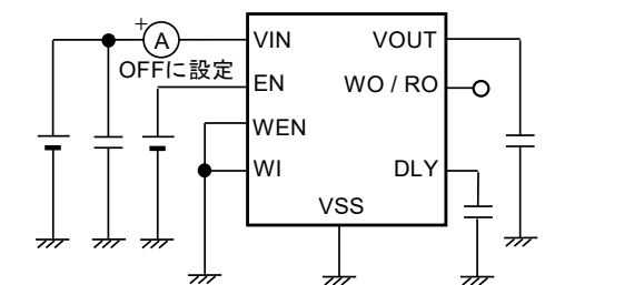
図22 測定回路10
