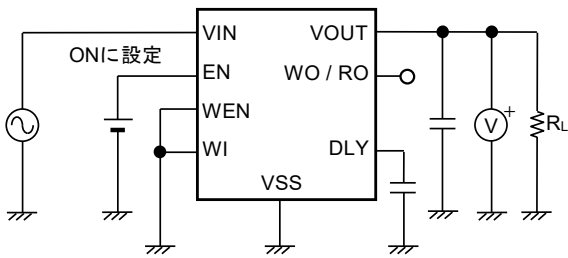
図15 測定回路3
