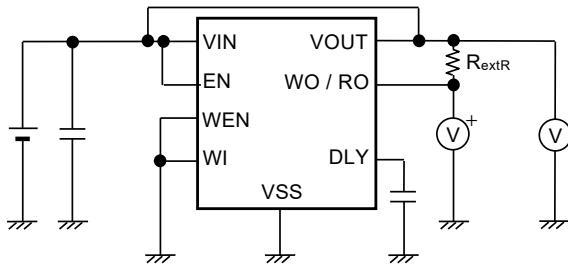
図17 測定回路5
