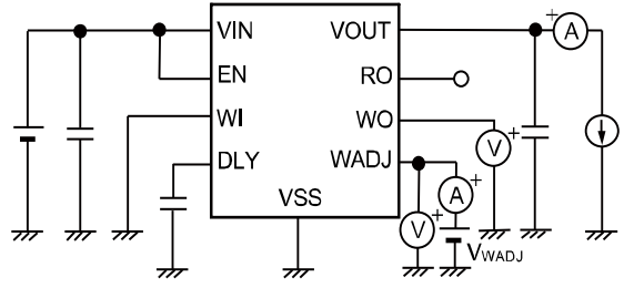
図30 測定回路8
