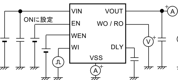
図21 測定回路9
