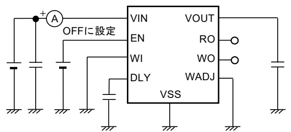
図32 測定回路10
