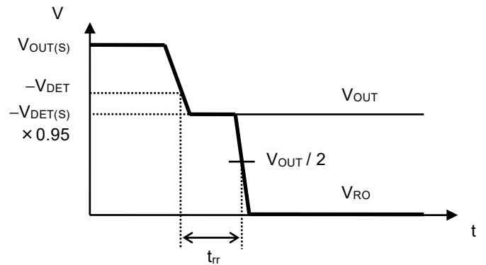
図8 リセット反応時間
