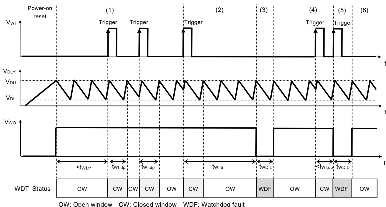
図41 ウォッチドッグタイマ部のタイミングチャート
