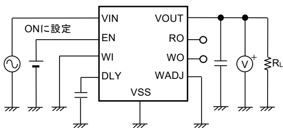
図25 測定回路3
