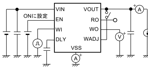
図31 測定回路9
