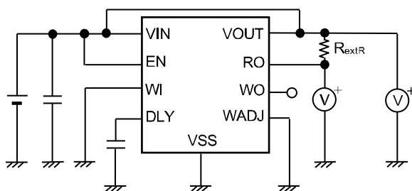
図27 測定回路5
