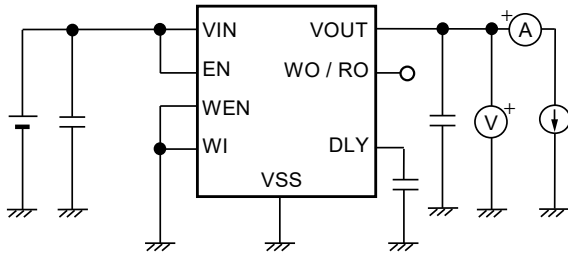
図13 測定回路1
