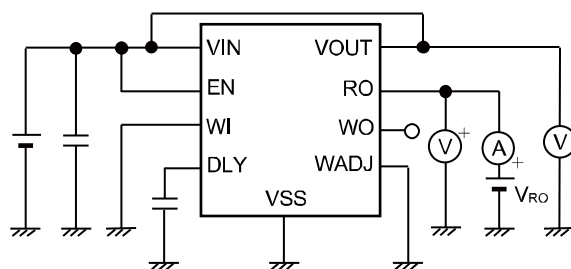
図28 測定回路6
