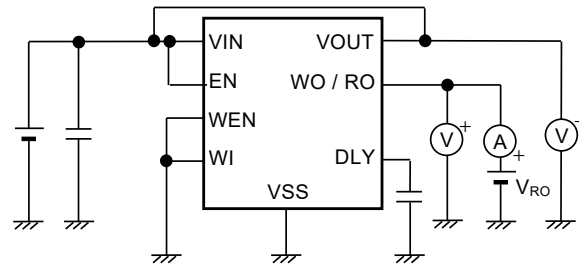
図18 測定回路6
