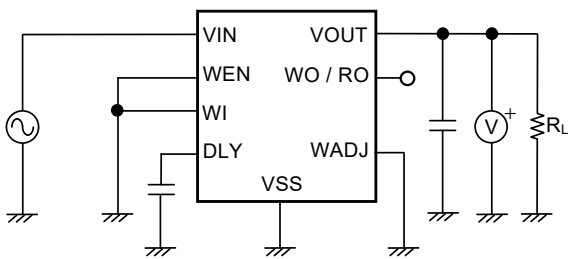
図14 測定回路3
