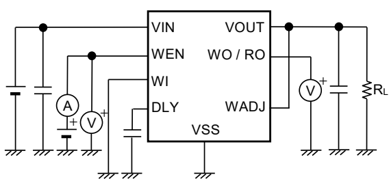
図20 測定回路9
