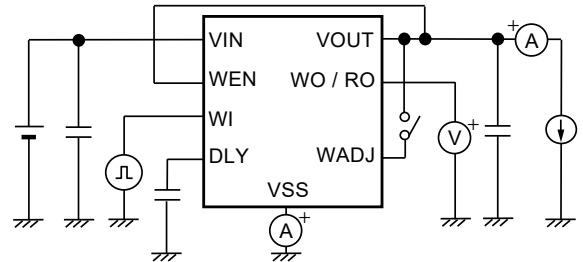
図21 測定回路10
