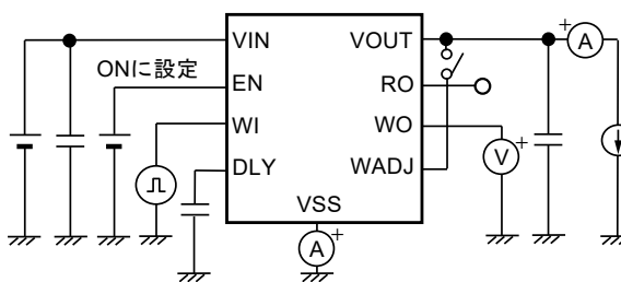
図29 測定回路9
