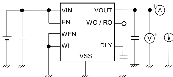
図11 測定回路1
