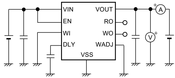
図22 測定回路2
