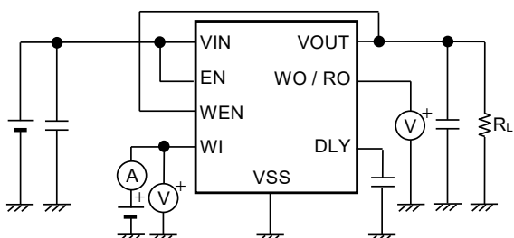
図17 測定回路7
