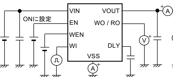
図19 測定回路9
