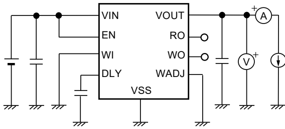
図21 測定回路1
