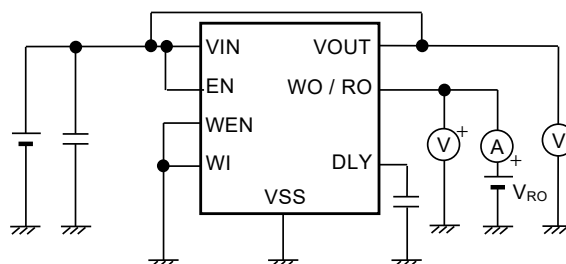
図16 測定回路6
