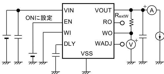
図27 測定回路7
