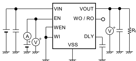
図14 測定回路4
