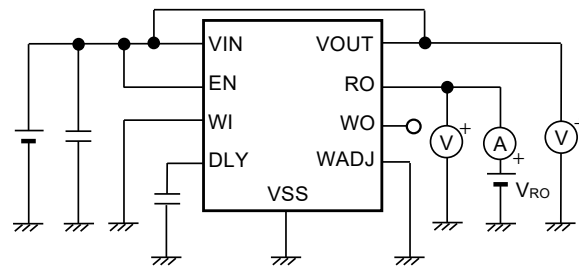
図26 測定回路6
