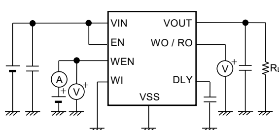
図18 測定回路8
