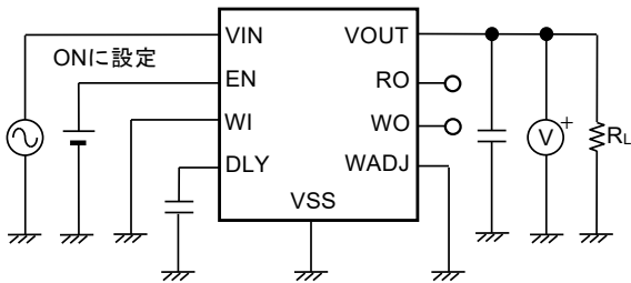
図23 測定回路3
