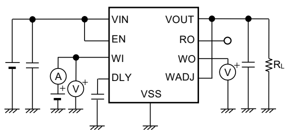
図31 測定回路11
