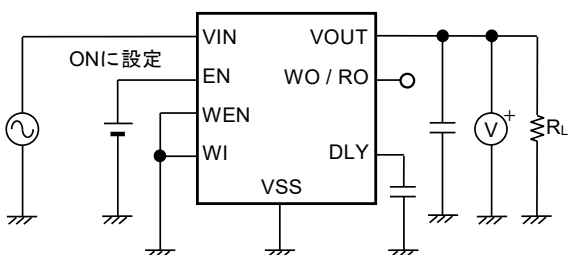
図13 測定回路3
