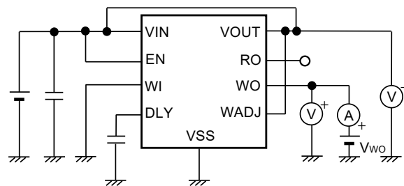
図32 測定回路12
