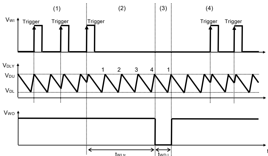
図39 ウォッチドッグタイマ部のタイミングチャート
