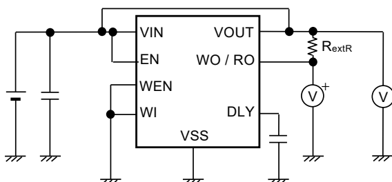
図15 測定回路5
