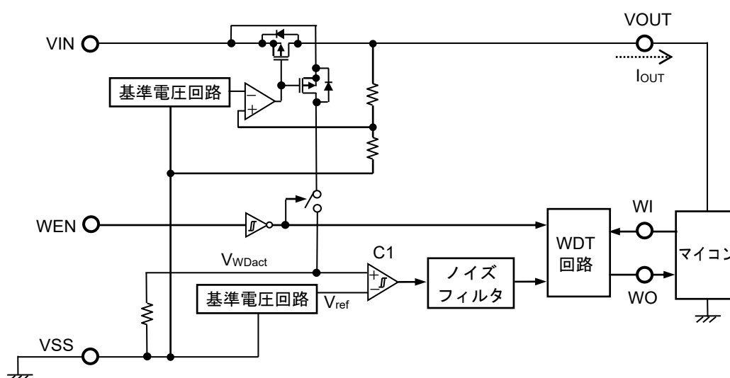
図41 出力電流検出回路の動作説明図
