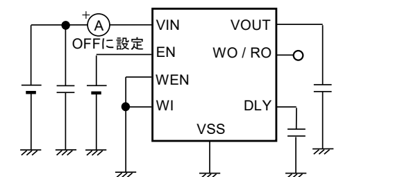
図20 測定回路10
