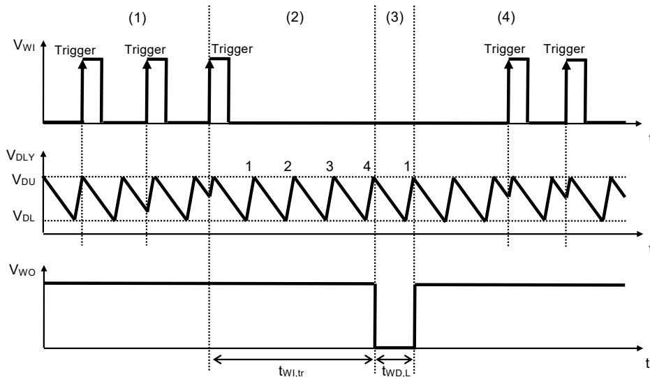
図43 ウォッチドッグタイマ部のタイミングチャート
