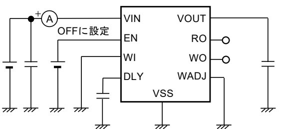
図30 測定回路10
