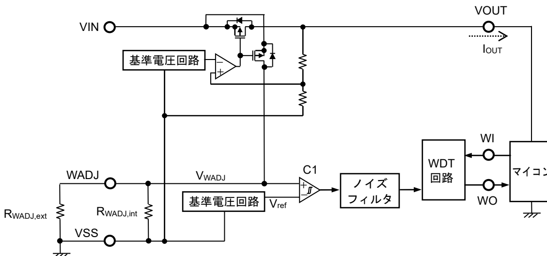
図45 出力電流検出回路の動作説明図
