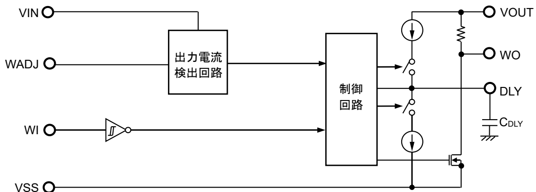
図44 ウォッチドッグタイマ部の動作説明図
