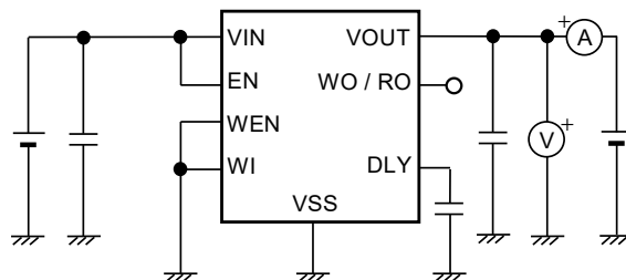
図12 測定回路2
