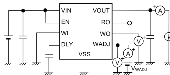
図28 測定回路8
