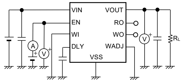
図24 測定回路4
