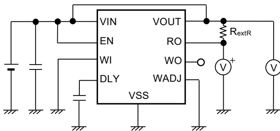
図25 測定回路5
