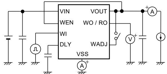
図19 測定回路10
