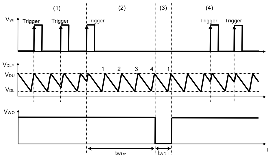
図35 ウォッチドッグタイマ部のタイミングチャート
