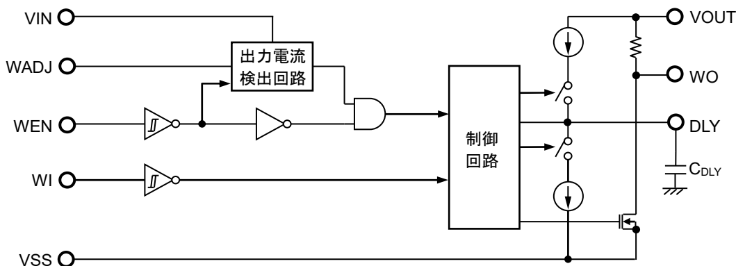
図36 ウォッチドッグタイマ部の動作説明図
