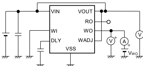
図28 測定回路9
