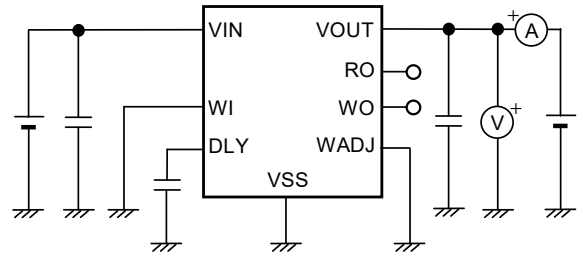
図21 測定回路2
