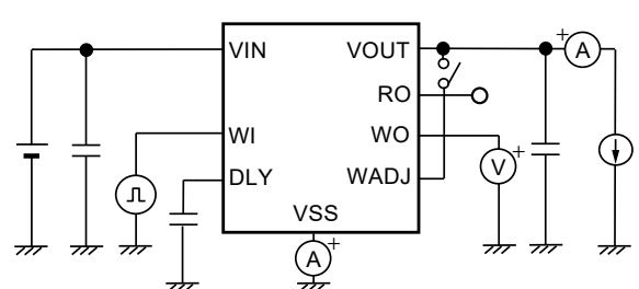
図29 測定回路10
