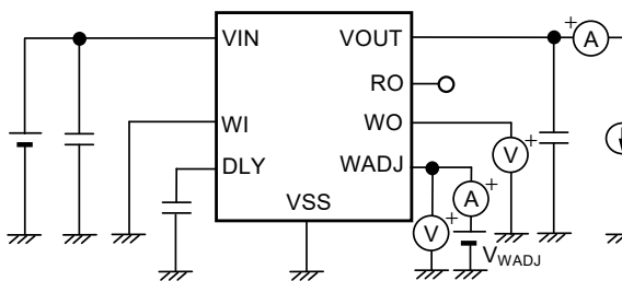
図26 測定回路7
