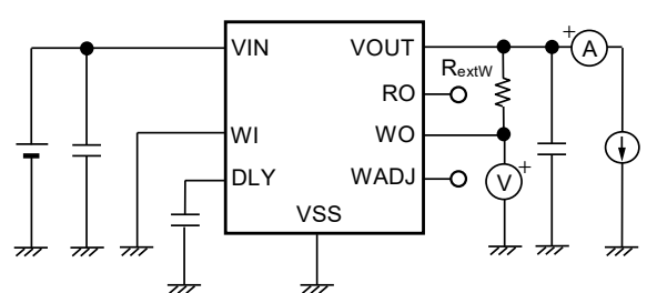
図25 測定回路6
