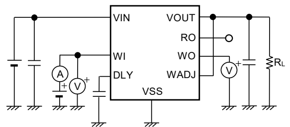
図27 測定回路8
