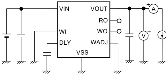
図20 測定回路1
