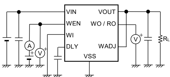
図18 測定回路9
