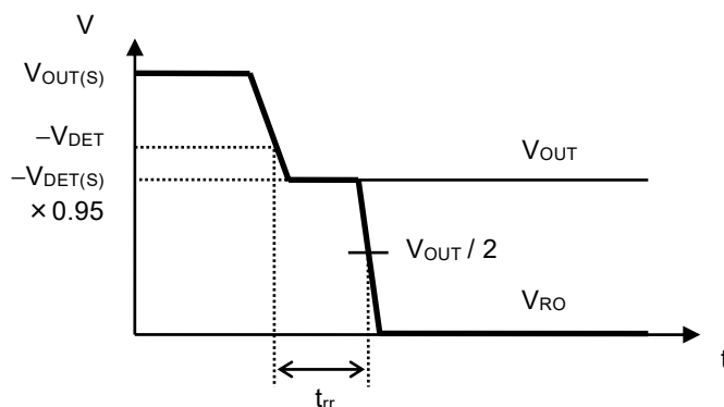
図7 リセット反応時間
