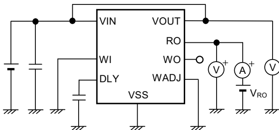
図24 測定回路5
