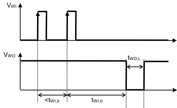
図9 ウォッチドッグトリガ時間
