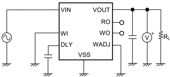
図22 測定回路3
