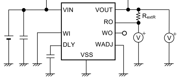
図23 測定回路4
