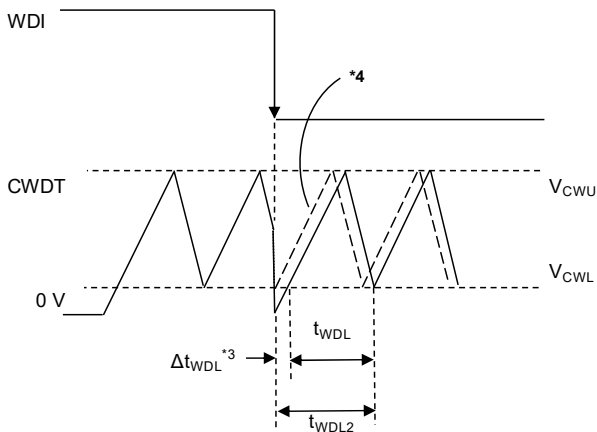
図15 V_{WDI} の立ち上がりエッジまたは立ち下がりエッジ
