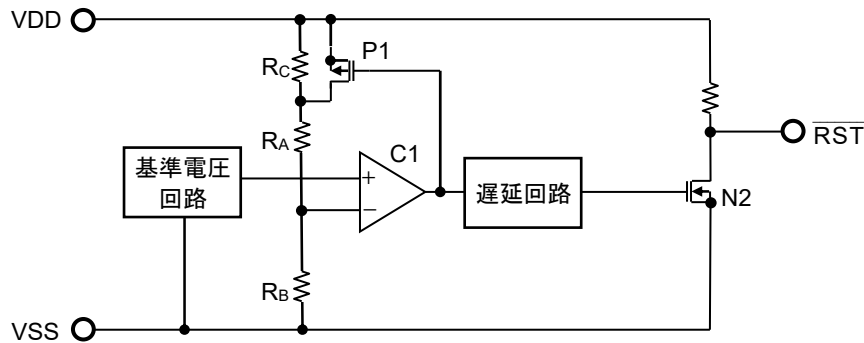
図31 電圧検出回路の動作説明図
