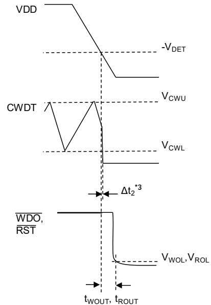
図10 CWDT端子充電動作中のV DD の立ち下がり
