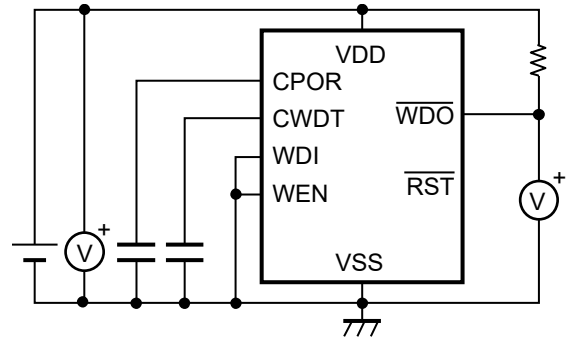
図16 測定回路1
