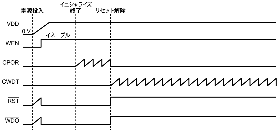
図35 WEN端子 = "H"
