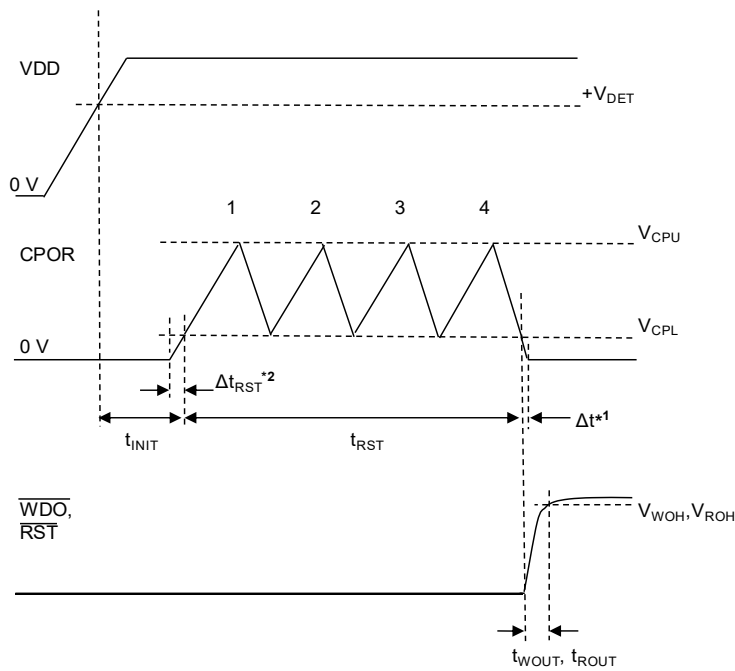
図8 V DD の立ち上がり
