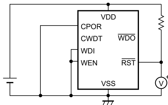
図20 測定回路5
