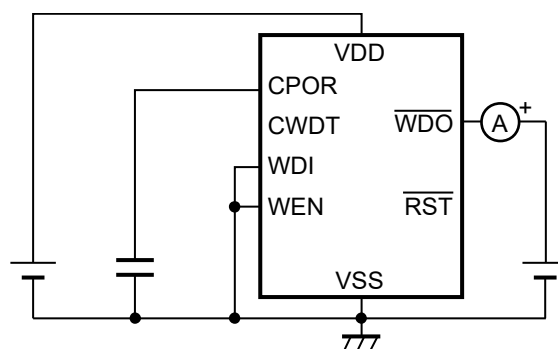
図26 測定回路11
