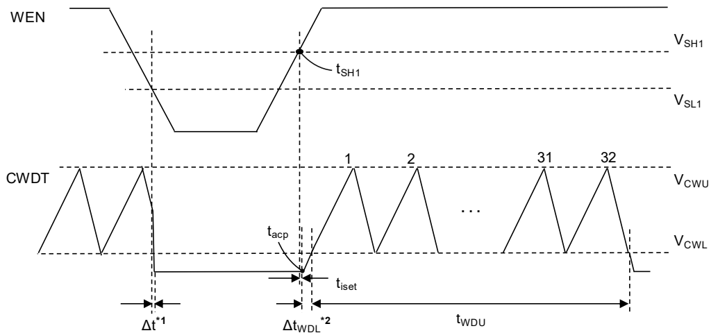
図11 V WEN によるカウンタリセット
