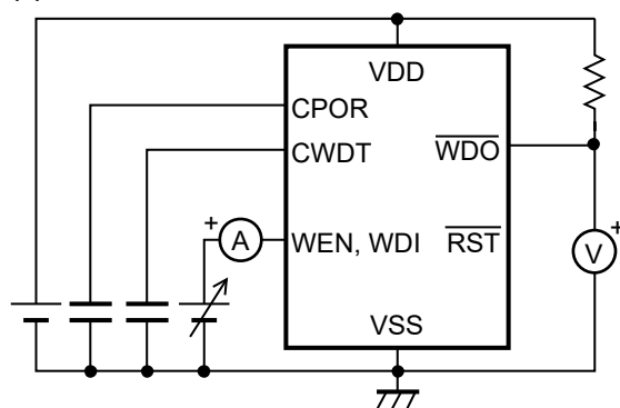
図27 測定回路12
