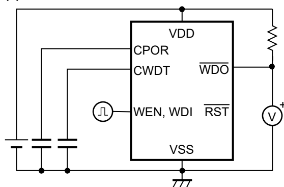
図28 測定回路13
