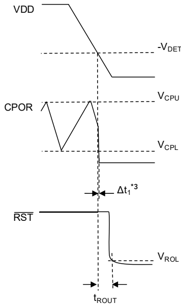
図9 CPOR端子充電動作中のV DD の立ち下がり
