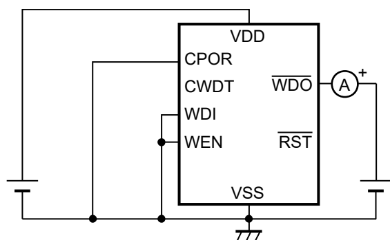
図25 測定回路10
