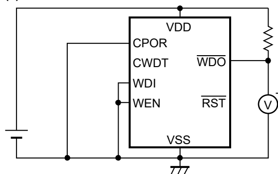
図24 測定回路9
