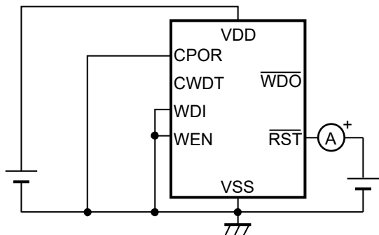
図21 測定回路6
