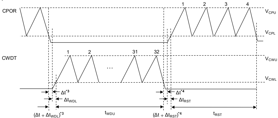
図12 ウォッチドッグタイムアウト検出
