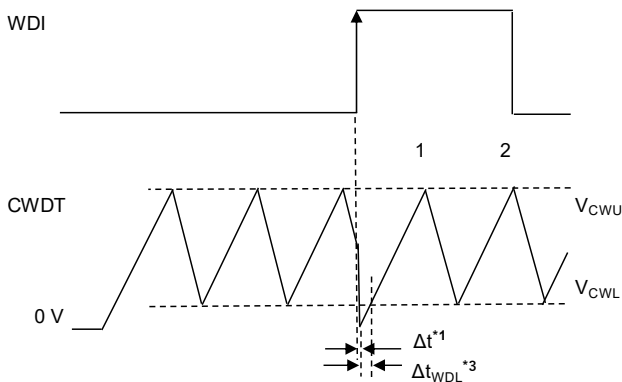
図13 V_{WDI} の立ち上がりエッジ
