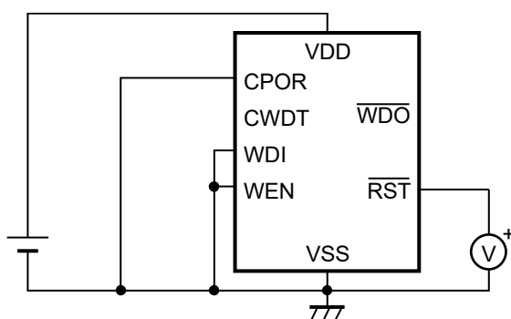
図19 測定回路4
