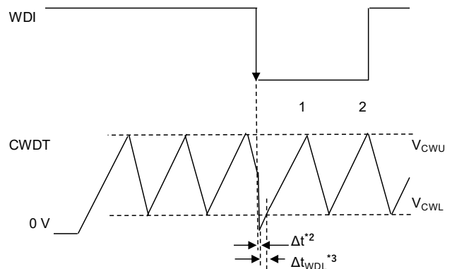
図14 V_{WDI} の立ち下がりエッジ
