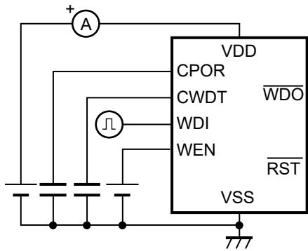
図17 測定回路2
