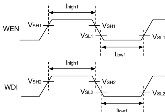
図7 入力パルス幅
