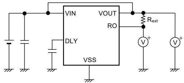
図9 測定回路4
