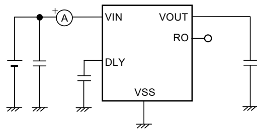
図11 測定回路6
