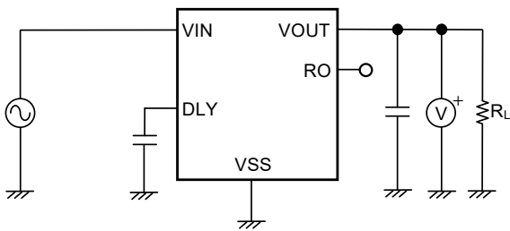
図8 測定回路3
