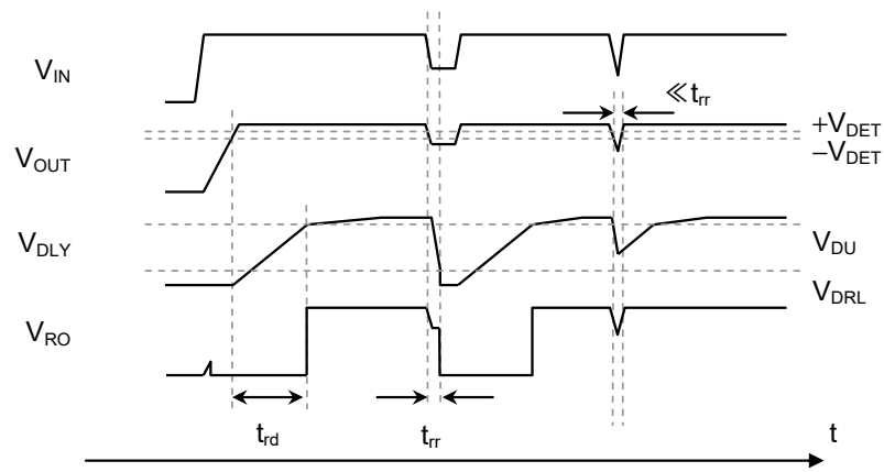
図16 ディテクタ動作例
