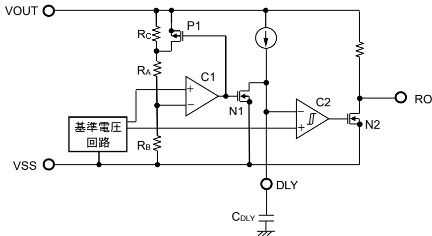
図14 ディテクタ部の動作説明図
