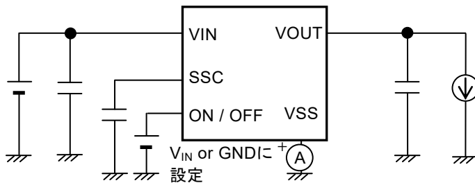
図4 測定回路2
