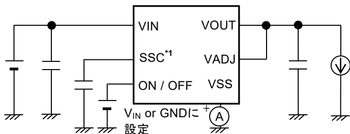
図17 測定回路9
