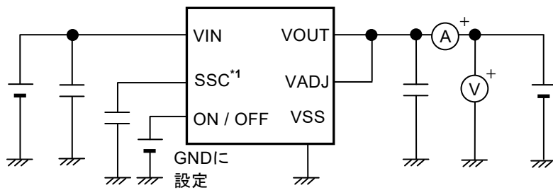
図21 測定回路13
