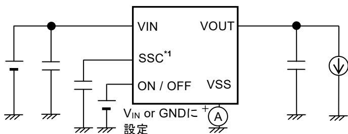
図10 測定回路2
