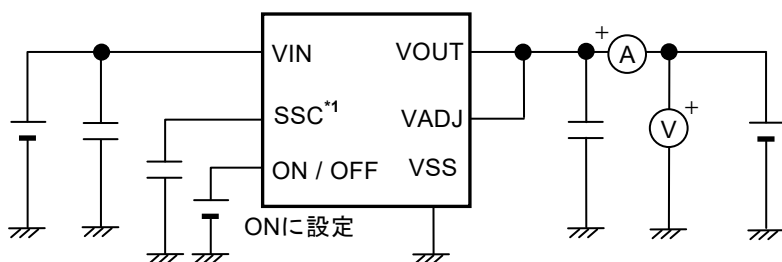
図18 測定回路10
