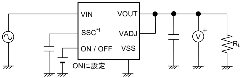
図20 測定回路12
