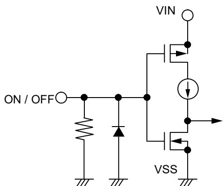
図29 S-19244xxxHシリーズ A / C / E / Gタイプ
