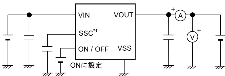
図11 測定回路3
