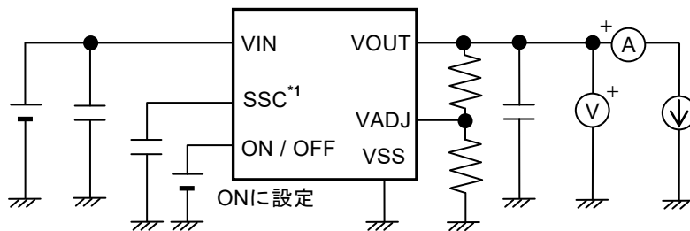
図23 測定回路15
