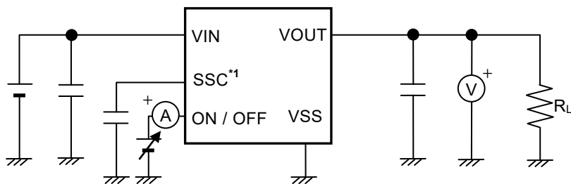
図12 測定回路4
