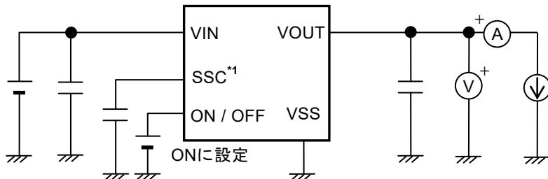
図9 測定回路1
