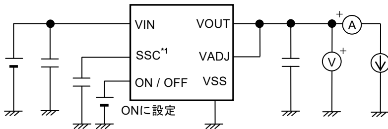
図16 測定回路8
