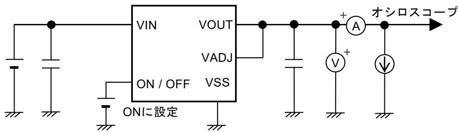
図22 測定回路14
