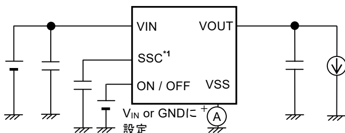
図10 測定回路2
