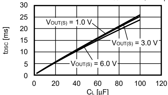
図34 S-19244xxxAシリーズA/Bタイプ (放電シャント機能あり)
