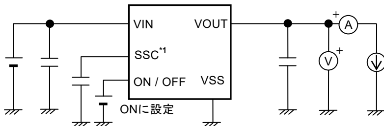
図9 測定回路1
