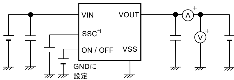
図14 測定回路6
