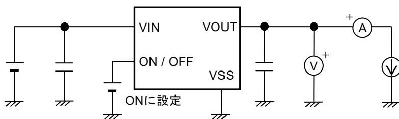
図8 測定回路1
