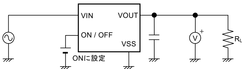
図12 測定回路5
