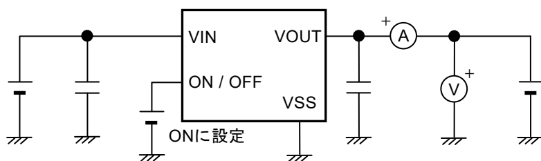
図10 測定回路3
