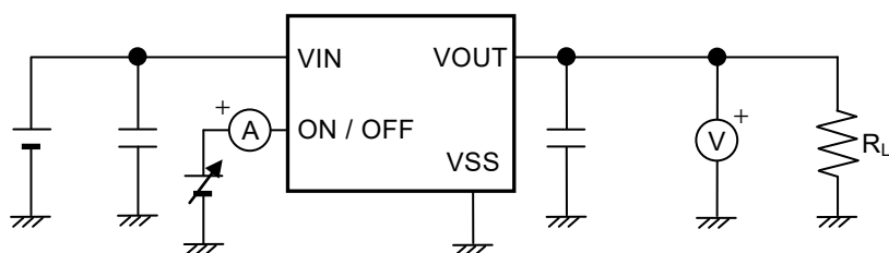
図11 測定回路4
