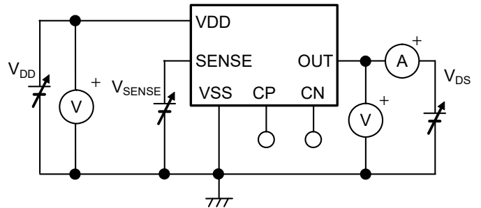
図14 測定回路3 (SENSE検出品)
