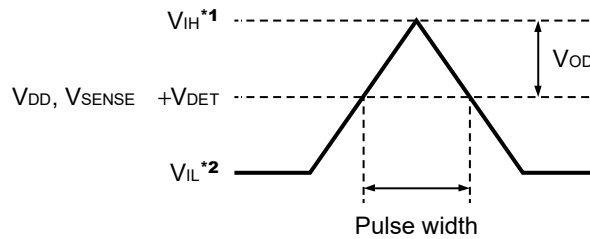
図50 VDD検出品
