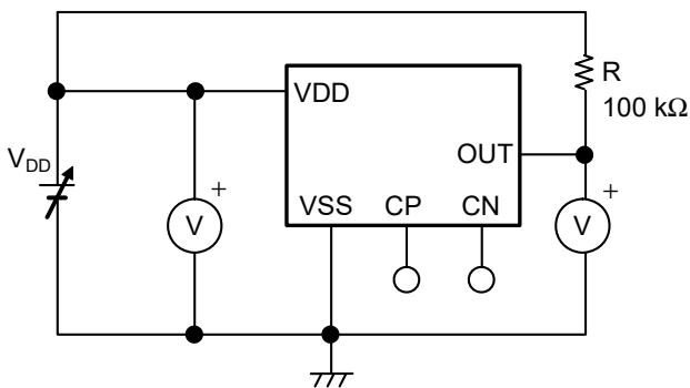
図23 検出電圧、解除電圧の測定回路 (VDD検出品)
