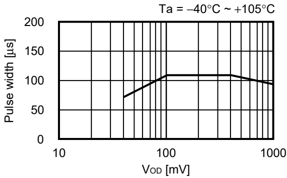
図50 VDD検出品
