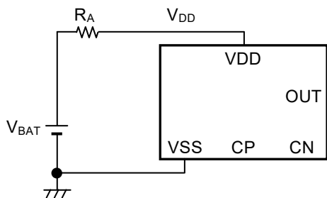
図42 VDD検出品
