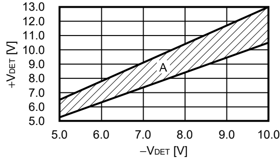
図5 検出電圧、解除電圧設定可能領域 ( -V_{DET} \leq 10.0\text{ V} )
