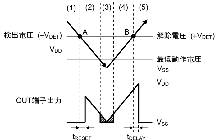
図31 S-19110シリーズDタイプの動作説明図
