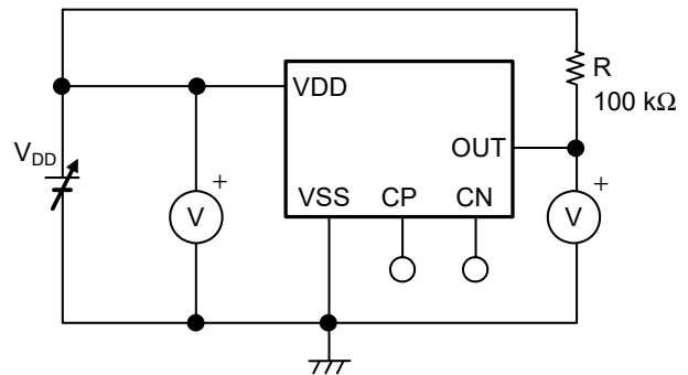
図69 ロードダンプ特性の測定回路
