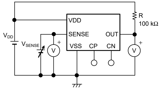
図10 測定回路1 (SENSE検出品)
