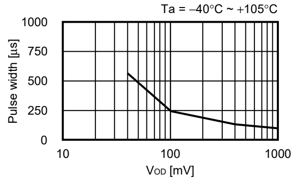
図51 SENSE検出品
