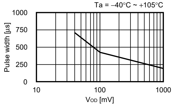
図48 SENSE検出品
