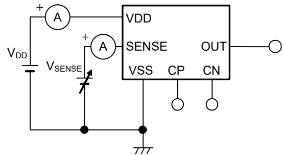
図12 測定回路2 (SENSE検出品)
