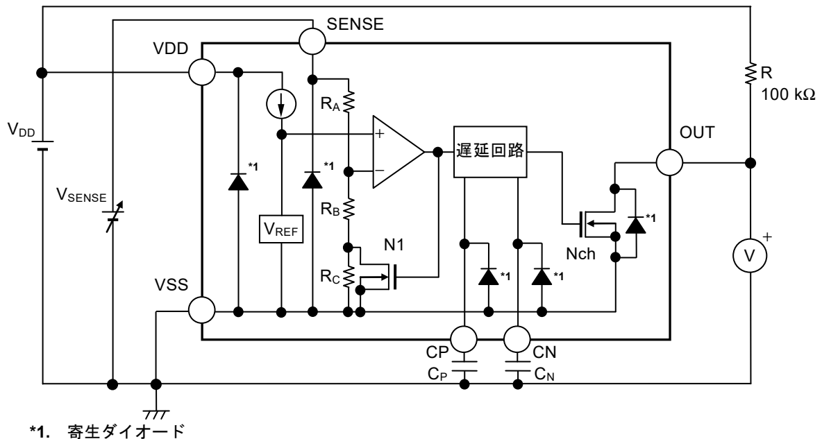
図33 S-19110シリーズEタイプの動作説明図
