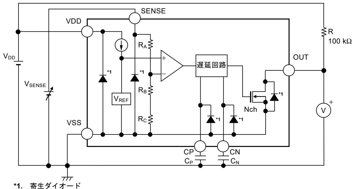
図37 S-19110シリーズGタイプの動作説明図
