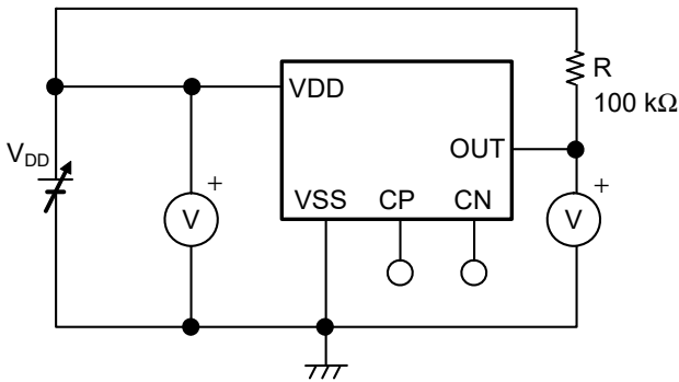
図9 測定回路1 (VDD検出品)
