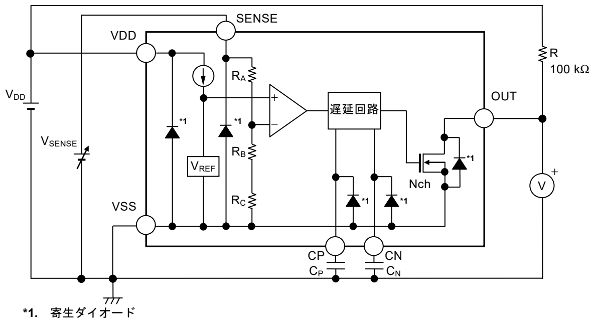
図39 S-19110シリーズHタイプの動作説明図
