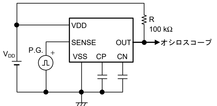
図16 測定回路4 (SENSE検出品)
