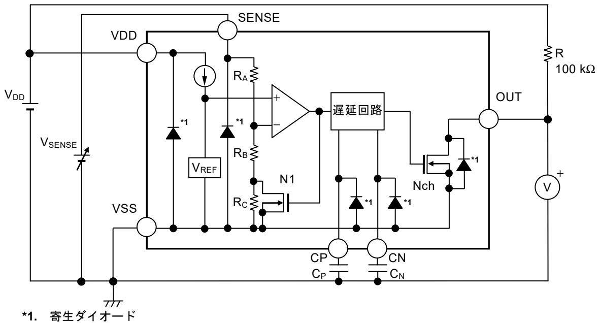
図35 S-19110シリーズFタイプの動作説明図
