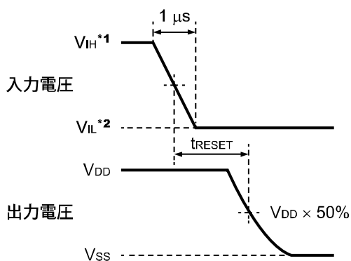
図61 検出遅延時間の測定条件
