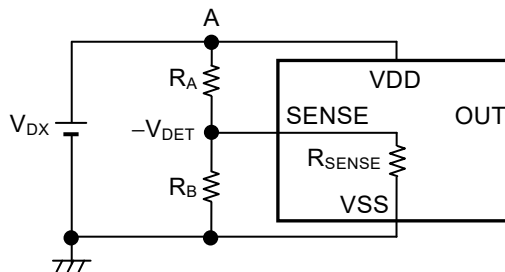
図23 検出電圧外部設定回路
