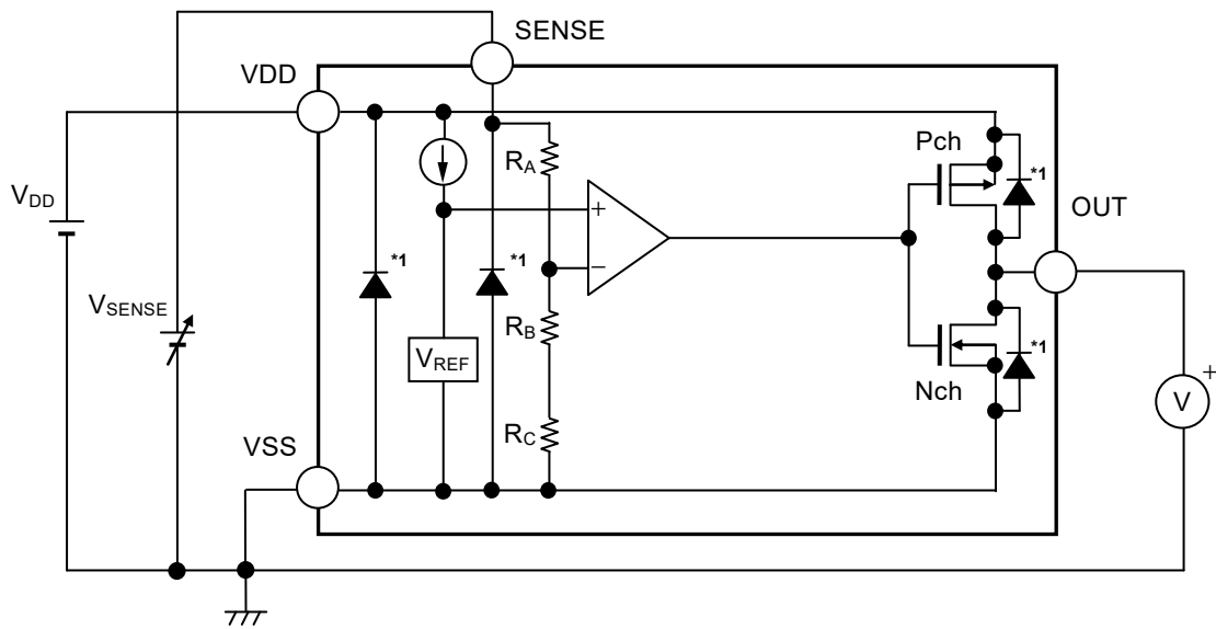
図21 S-19103/19109シリーズCタイプの動作説明図
