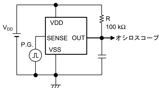
図30 応答時間の測定回路 (Nchオープンドレイン出力品)
