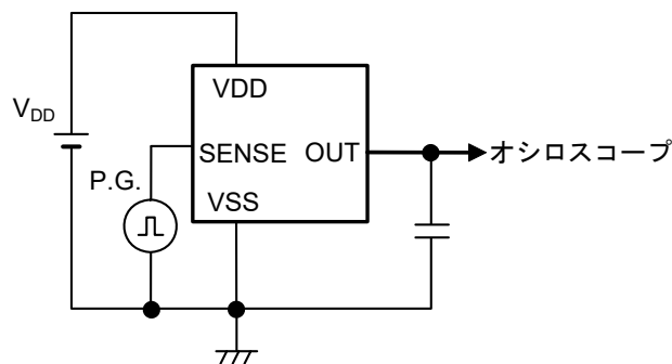
図31 応答時間の測定回路 (CMOS出力品)
