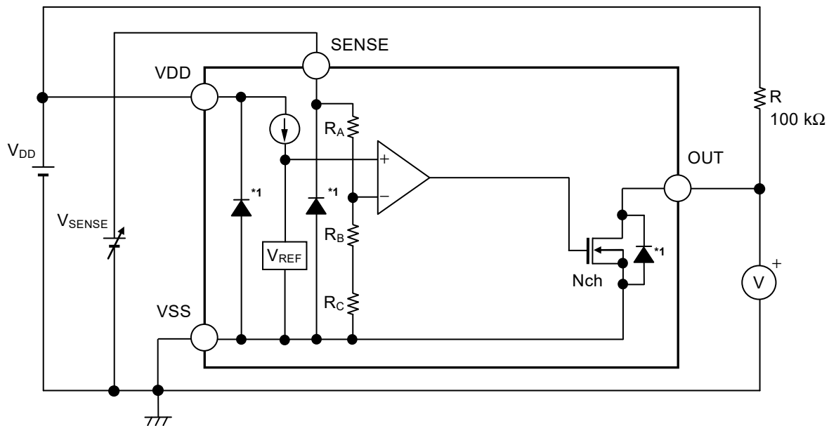
図19 S-19103/19109シリーズNタイプの動作説明図
