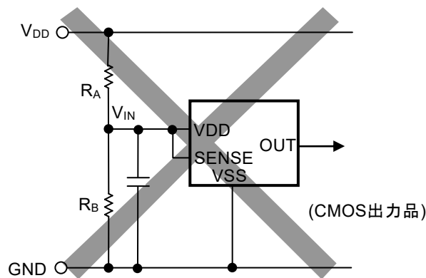
図18 検出電圧変更回路不良事例
