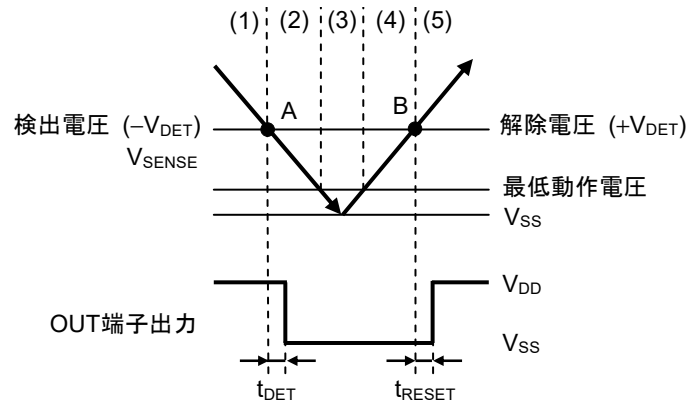
図20 S-19103/19109シリーズNタイプのタイミングチャート
