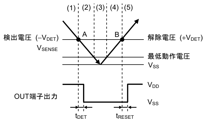
図21 S-19103/19109シリーズCタイプの動作説明図
