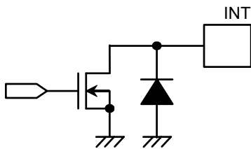
図7 INT端子 (Nchオープンドレイン出力)
