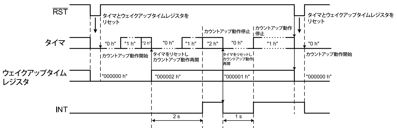
図19 ハンドシェイクタイムアウトの出力タイミング例 (CMOS出力)
