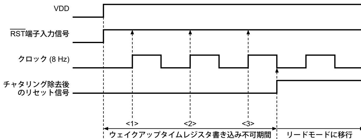
図35 電源投入時のタイミングチャート
