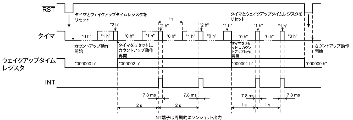
図13 ワンショットループタイムアウトの出力タイミング例 (CMOS出力)
