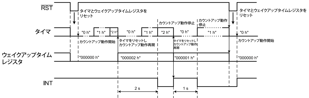
図18 ハンドシェイクタイムアウトの出力タイミング例 (Nchオープンドレイン出力)
