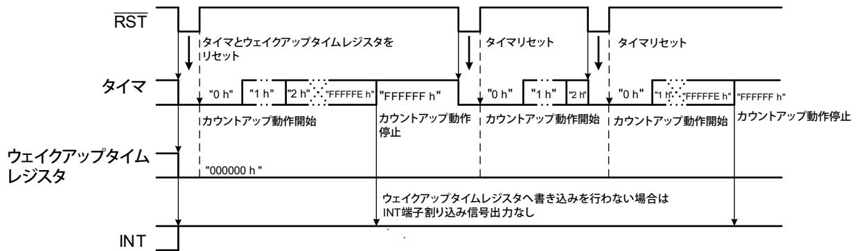
図14 ウェイクアップタイムレジスタに書き込みを行わない場合 (Nchオープンドレイン出力)
