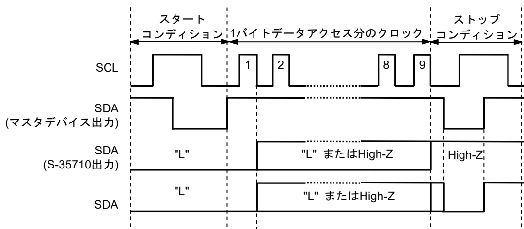
図30 SDAの解放方法
