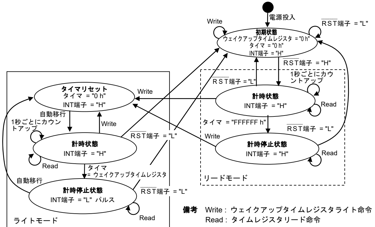
図16 ワンショットループタイムアウトの状態遷移図 (Nchオープンドレイン出力)
