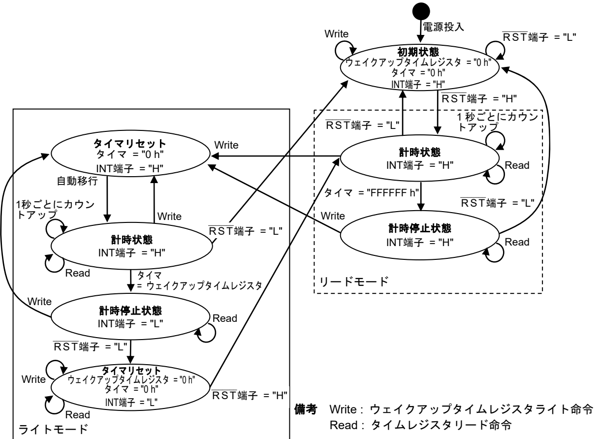
図20 ハンドシェイクタイムアウトの状態遷移図 (Nchオープンドレイン出力)
