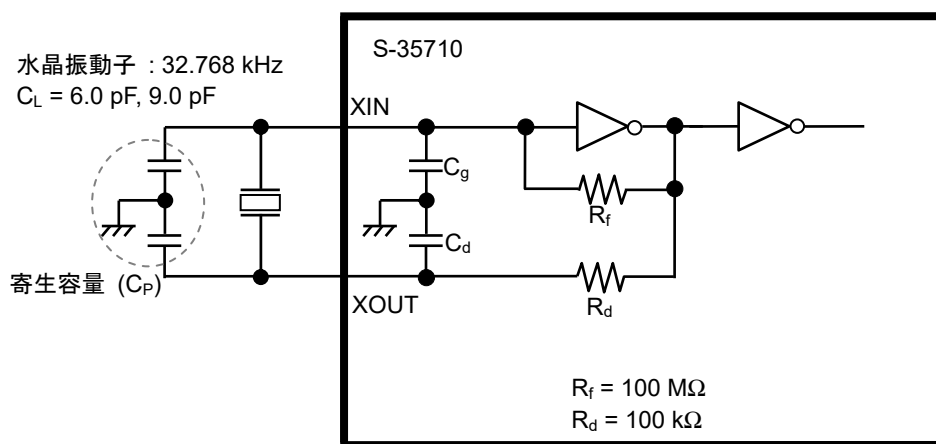
図37 水晶発振回路構成
