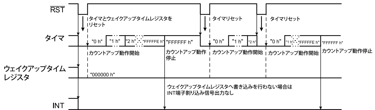
図15 ウェイクアップタイムレジスタに書き込みを行わない場合 (CMOS出力)
