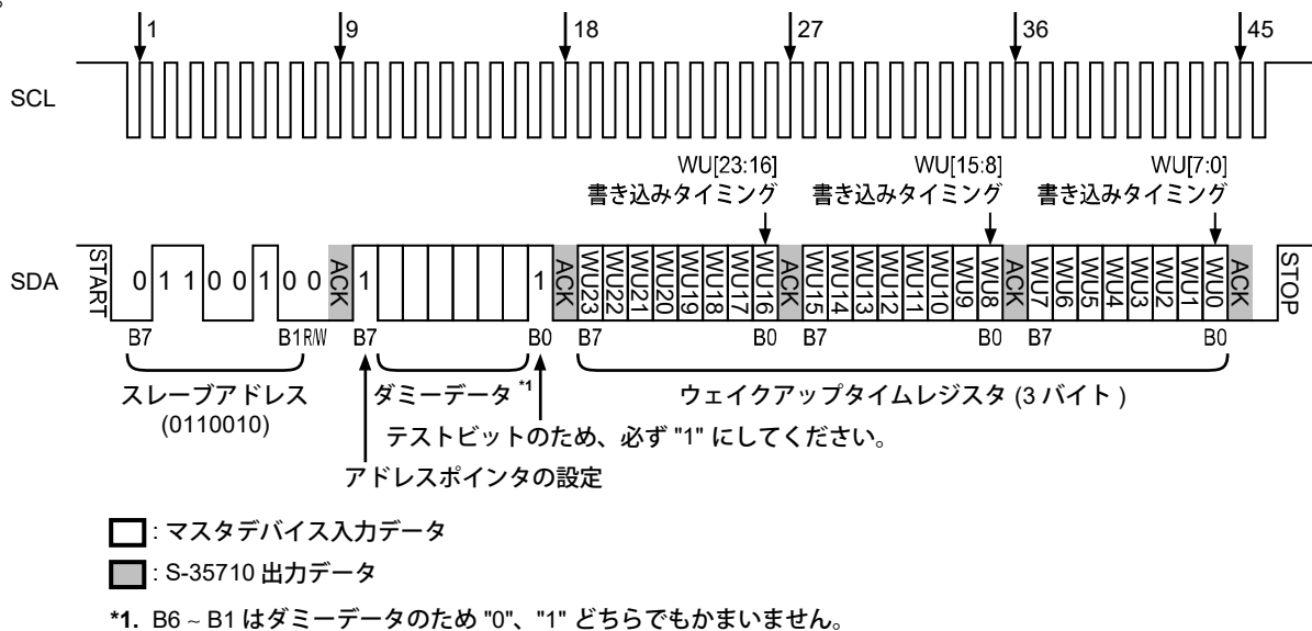
図28 ウェイクアップタイムレジスタの書き込みタイミング
