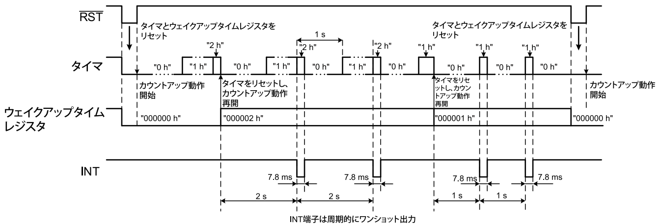
図12 ワンショットループタイムアウトの出力タイミング例 (Nchオープンドレイン出力)
