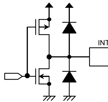
図8 INT端子 (CMOS出力)
