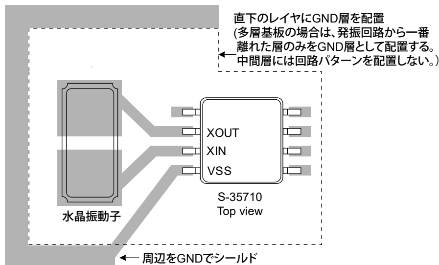
図38 接続パターン図の推奨例
