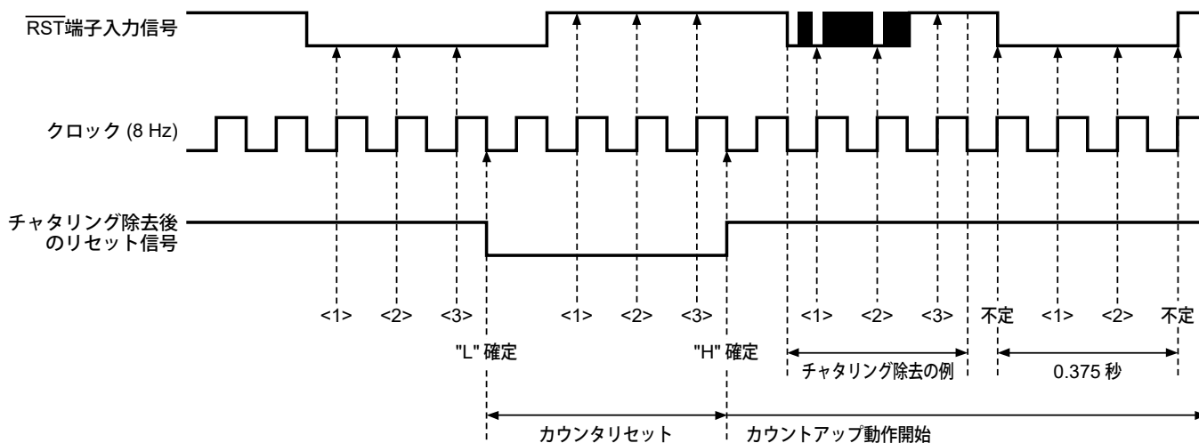
図34 チャタリング除去のタイミングチャート例
