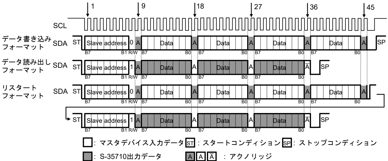
図26 シリアルインタフェースのデータ転送フォーマット
