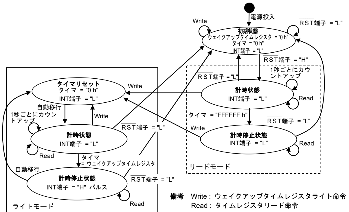
図17 ワンショットループタイムアウトの状態遷移図 (CMOS出力)
