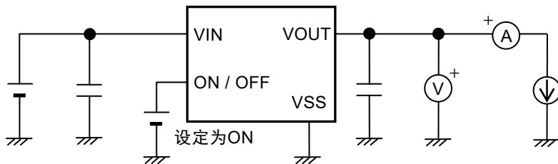
图8 测定电路1
