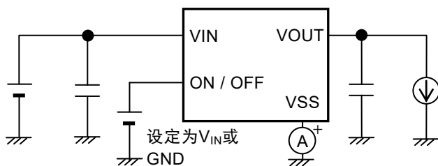
图9 测定电路2
