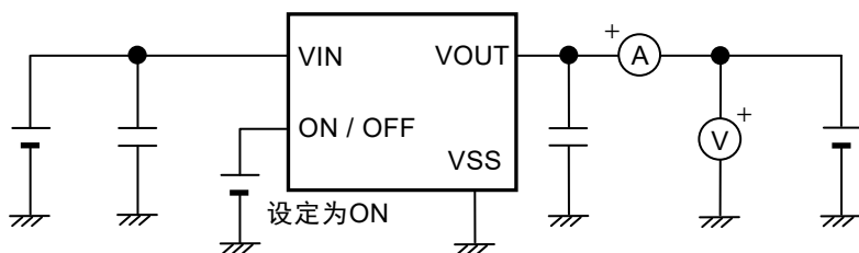
图10 测定电路3
