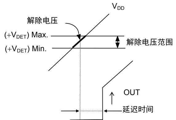
图15 解除电压
