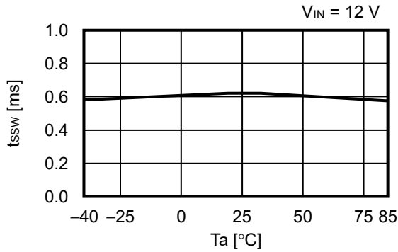
2.7 软启动等待时间 ( t_{SSW} ) – 温度 ( T_a )
