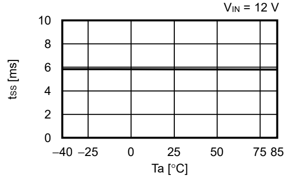
2.8 软启动时间 ( t_{SS} ) – 温度 ( T_a )
