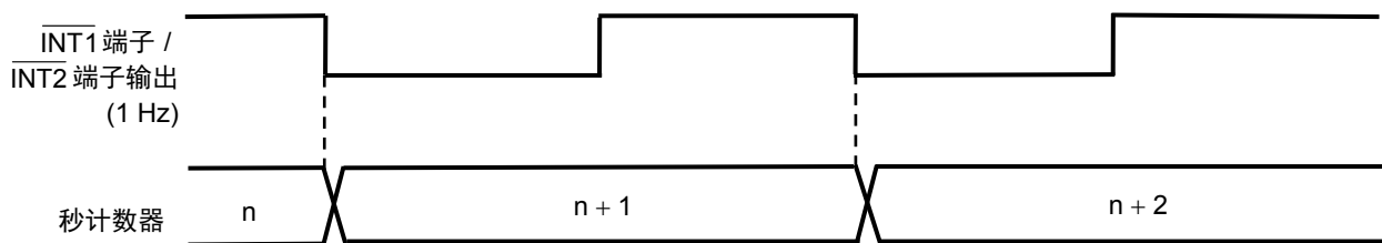
图17 1 Hz的时钟输出和秒计数器
