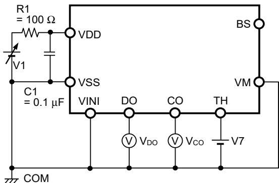
图3 测定电路1
