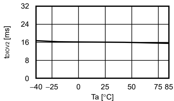
3.6 t_{dIOV2} - T_a
