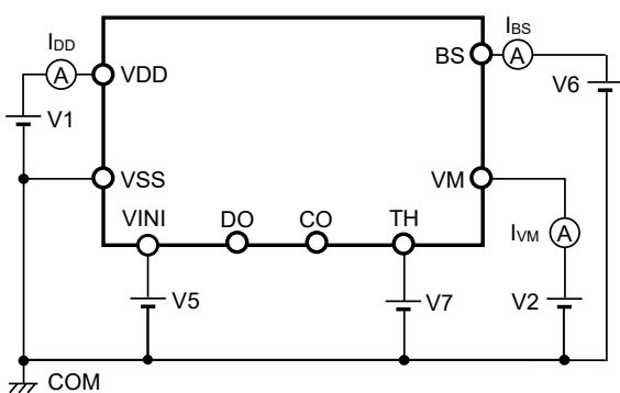
图5 测定电路3
