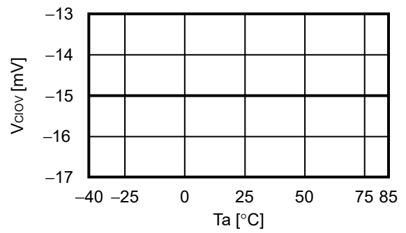
2.12 V_{CLOV} - T_a
