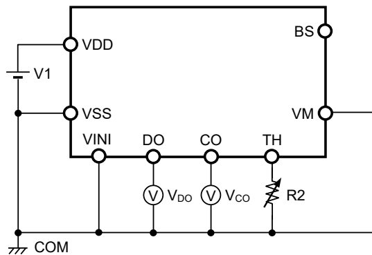
图8 测定电路6
