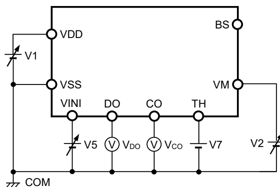
图4 测定电路2
