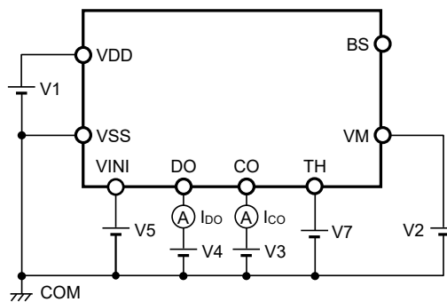
图6 测定电路4
