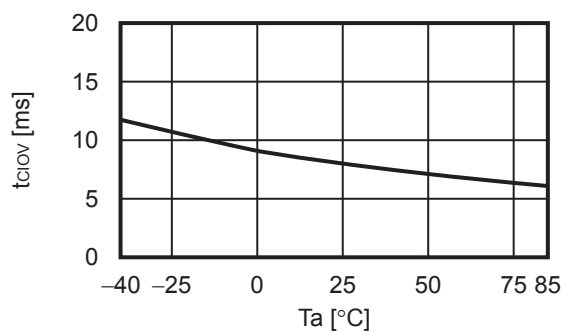
3.8 t_{CIOV} - T_a
