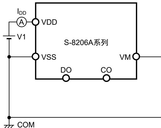
图8 测定电路2
