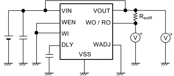
图13 测定电路4
