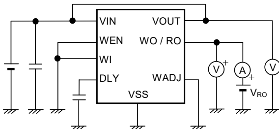
图14 测定电路5
