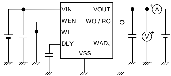
图11 测定电路2
