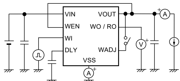
图19 测定电路10
