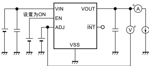
图7 测定电路1
