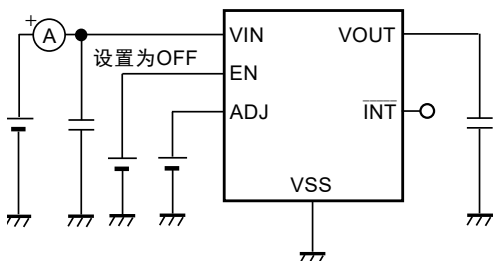
图11 测定电路5
