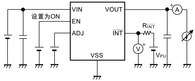
图16 测定电路10
