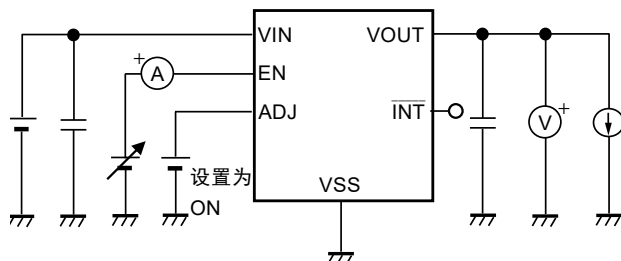
图12 测定电路6
