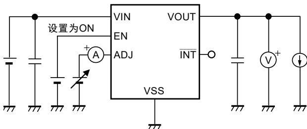
图13 测定电路7
