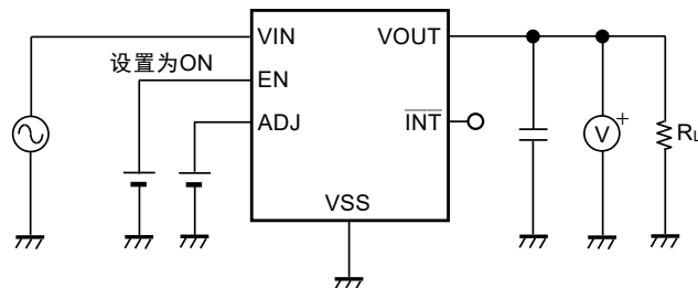
图14 测定电路8
