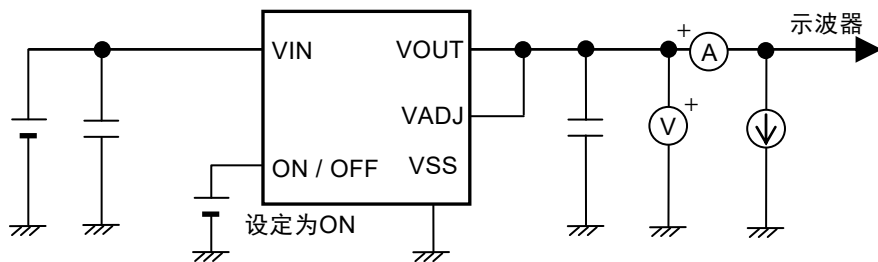
图22 测定电路14
