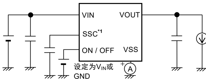
图10 测定电路2
