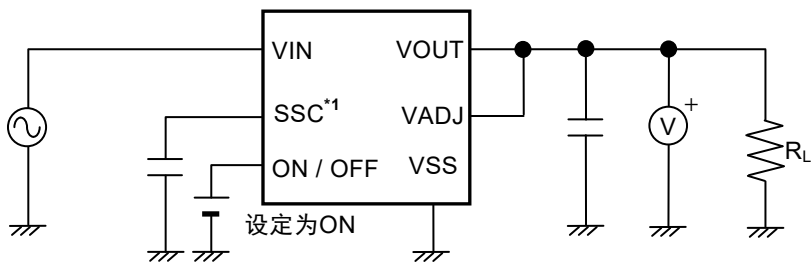
图20 测定电路12
