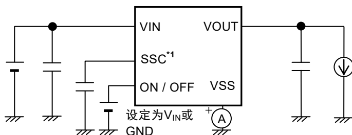
图10 测定电路2
