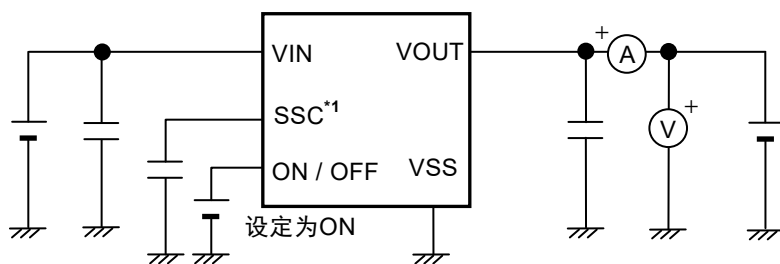
图11 测定电路3
