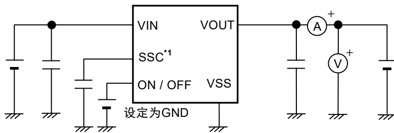
图14 测定电路6
