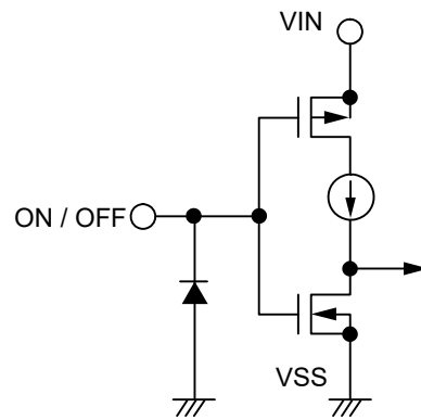
图30 S-19244xxxA系列B / D / F / H型
