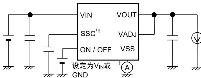
图17 测定电路9
