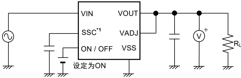
图20 测定电路12
