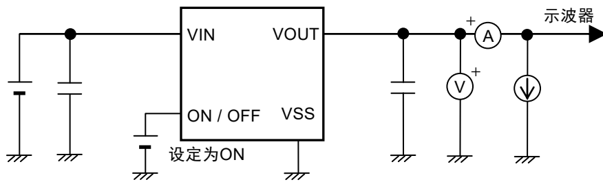
图15 测定电路7
