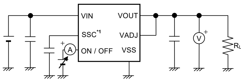
图19 测定电路11
