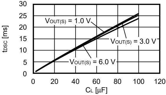
图34 S-19244xxxA系列A/B型 (有放电分路功能)
