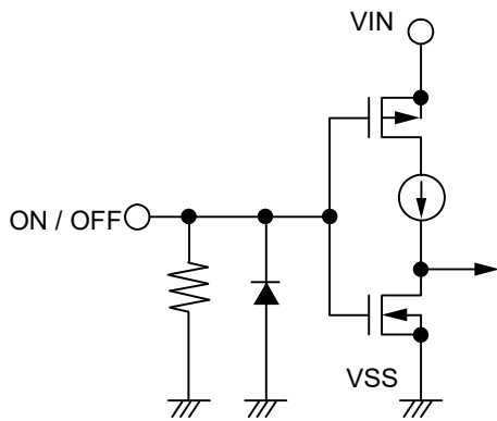
图29 S-19244xxxA系列A / C / E / G型
