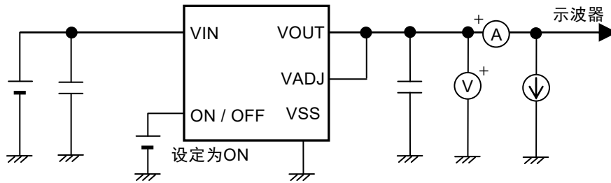
图22 测定电路14
