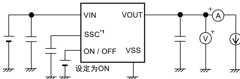
图9 测定电路1
