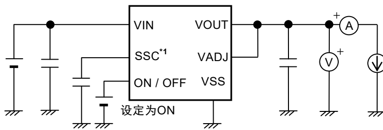
图16 测定电路8
