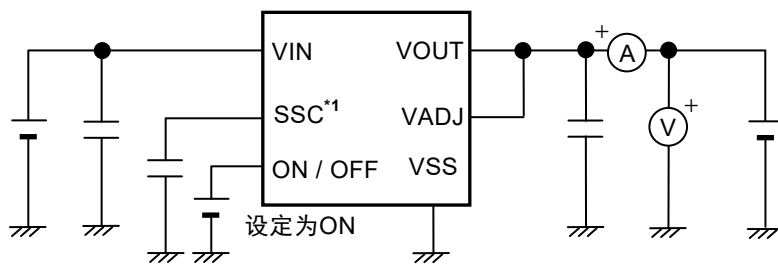
图18 测定电路10
