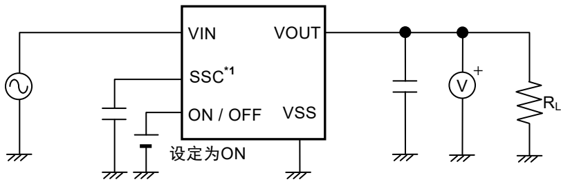
图13 测定电路5
