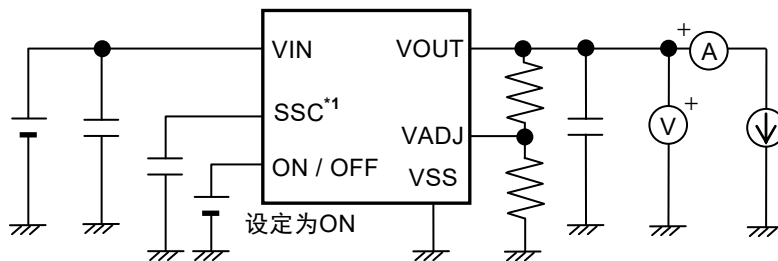
图23 测定电路15
