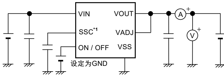
图21 测定电路13
