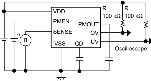
图7 测定电路3
