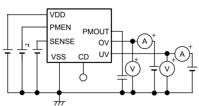
图6 测定电路2
