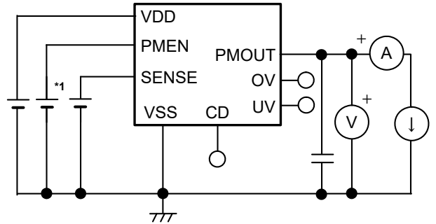
图8 测定电路4
