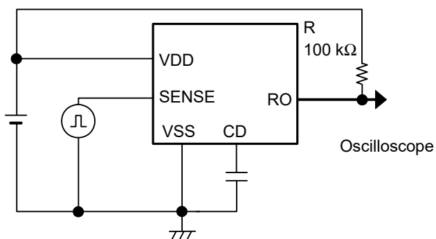
图9 测定电路3
