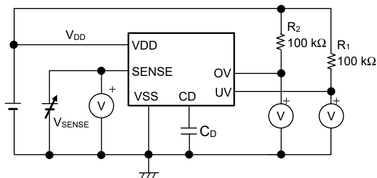
图22 HSNT-8(1616)B的检测电压、解除电压的测定电路
