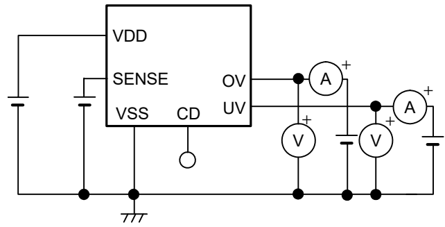
图12 测定电路6
