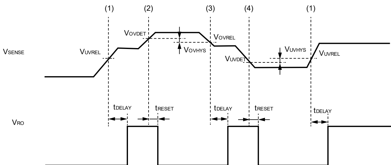
图26 时序
