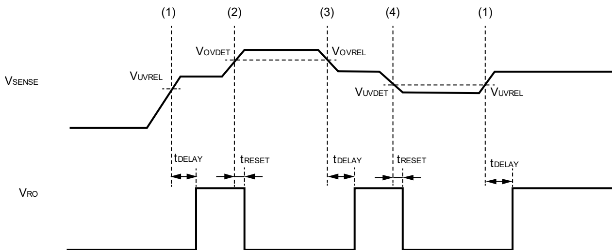
图24 时序
