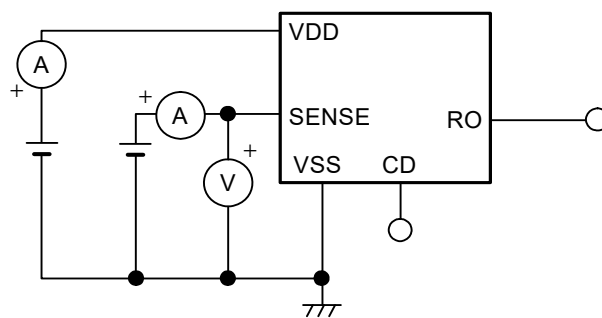
图10 测定电路4
