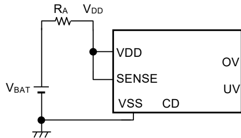
图34 HSNT-8(1616)B脚
