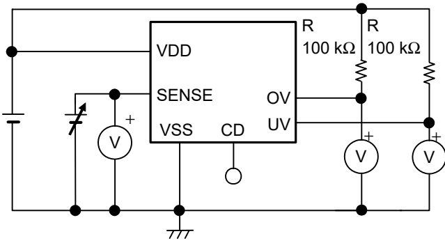
图11 测定电路5
