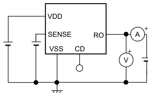
图8 测定电路2
