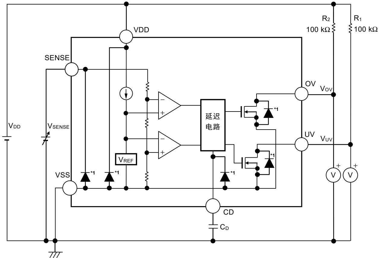
图27 工作说明
