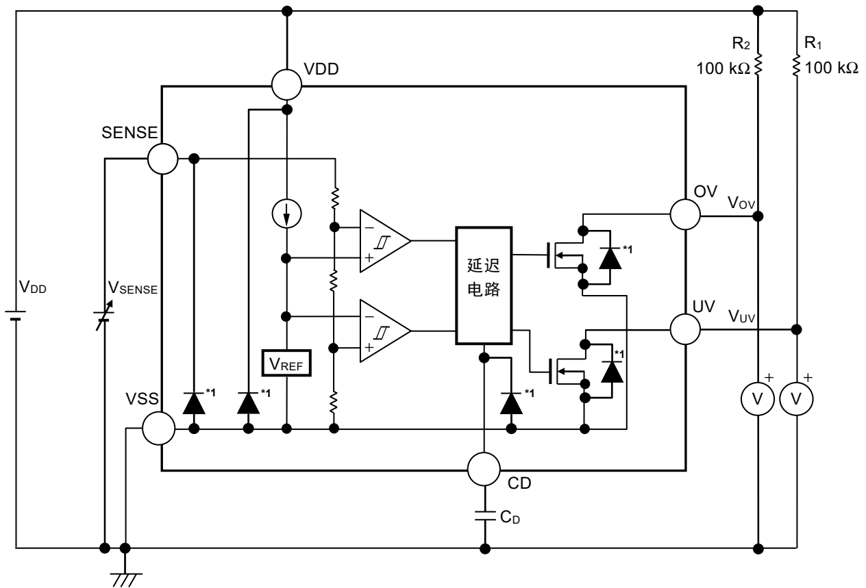
图29 工作说明
