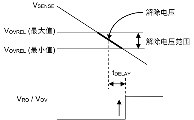
图18 过压解除电压
