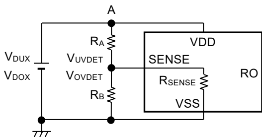
图31 SOT-23-6的检测电压外部设定电路
