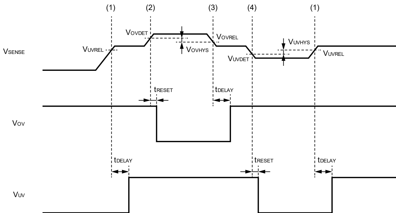
图30 时序
