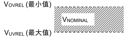
图36 V_{NOMINAL} > 0
