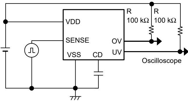
图13 测定电路7
