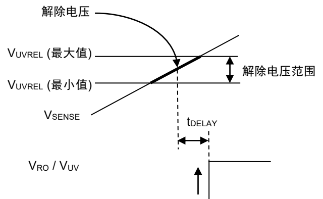
图20 欠压解除电压
