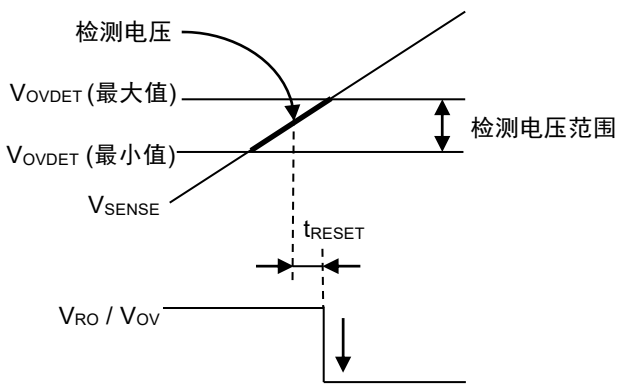
图17 过压检测电压
