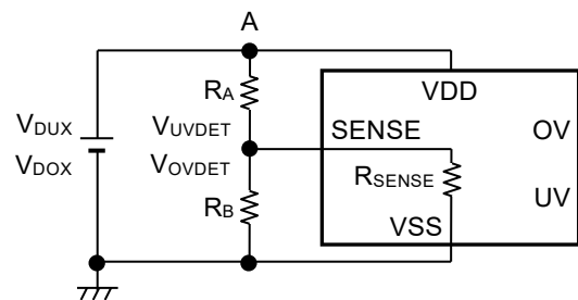
图32 HSNT-8(1616)B的检测电压外部设定电路
