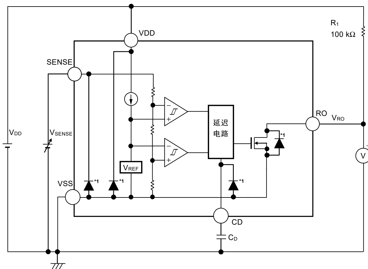
图25 工作说明
