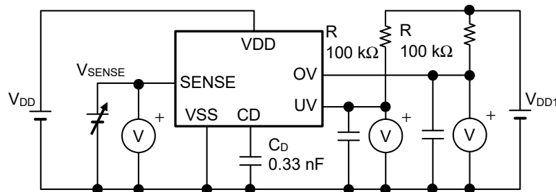
图40 响应时间的测定电路
