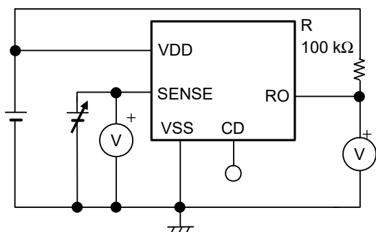
图7 测定电路1
