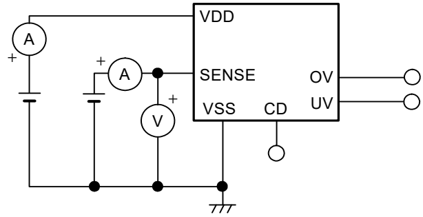
图14 测定电路8
