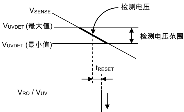
图19 欠压检测电压
