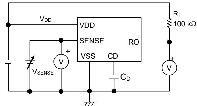
图21 SOT-23-6的检测电压、解除电压的测定电路
