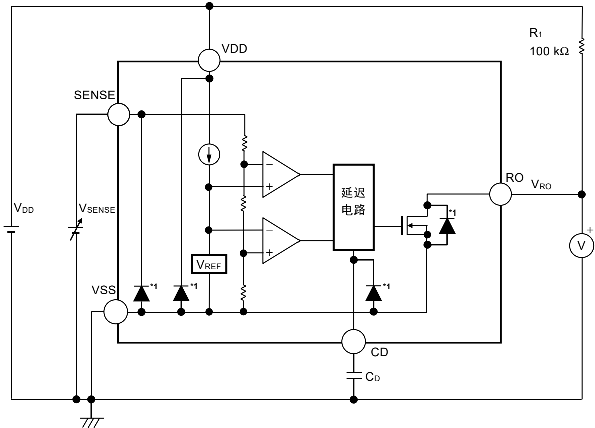
图23 工作说明
