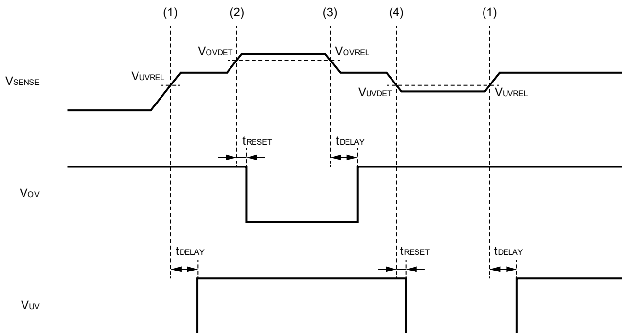
图28 时序
