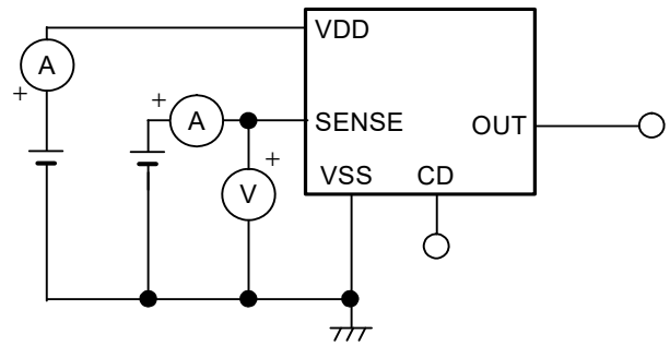
图9 测定电路4
