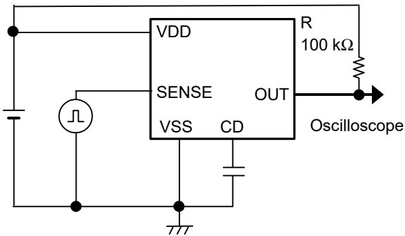
图8 测定电路3
