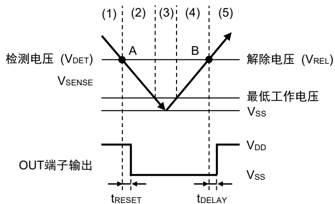
图15 S-19113系列L型的时序
