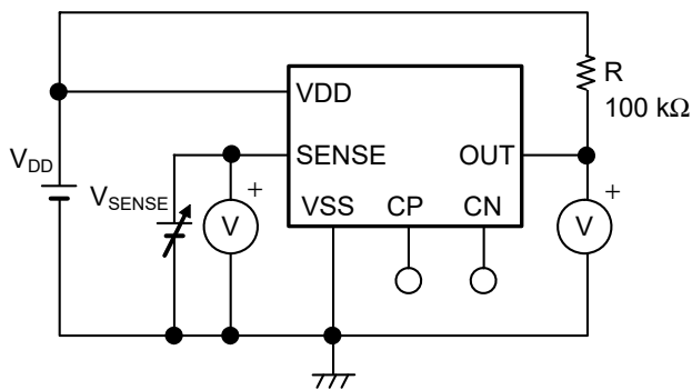
图24 检测电压、解除电压的测定电路 (SENSE检测产品)
