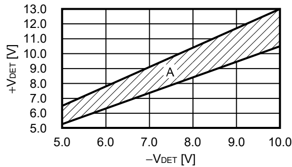
图5 检测电压、解除电压可设领域 ( -V_{DET} \leq 10.0\text{ V} )
