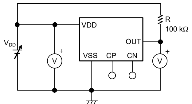
图69 抛负载特性的测定电路
