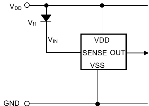
图37 使用二极管后检测电压的改变 (CMOS输出产品)
