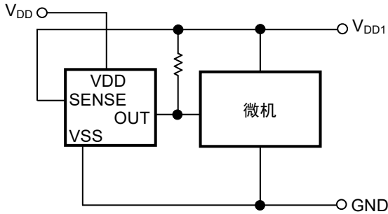
图32 复位电路示例 (N沟道开路漏极输出产品)
