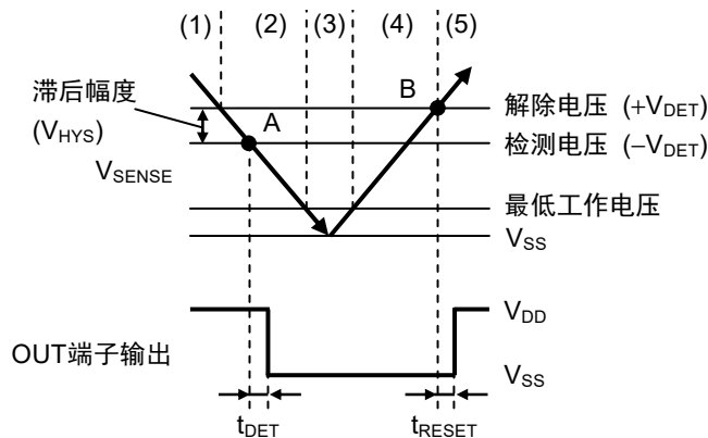
图20 S-19102/19108系列N型的时序图
