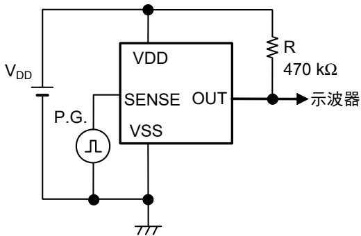
图9 测定电路4 (N沟道开路漏极输出产品)
