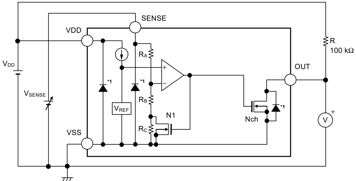
图19 S-19102/19108系列N型的工作说明图
