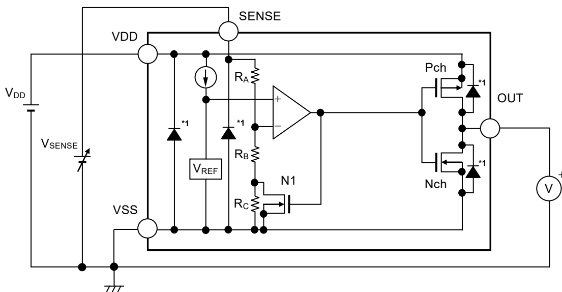
图21 S-19102/19108系列C型的工作说明图
