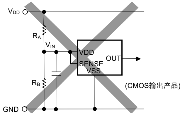
图18 检测电压改变电路不良事例
