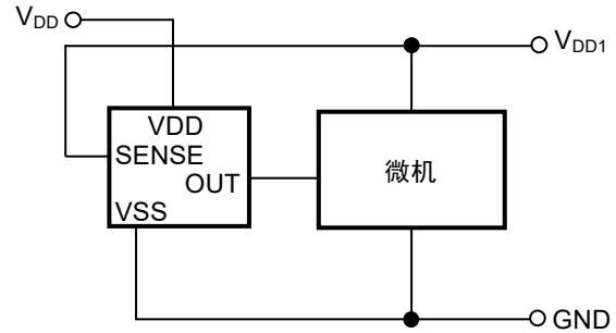
图33 复位电路示例 (CMOS输出产品)
