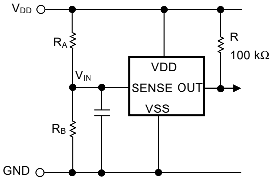
图34 使用分割电阻后检测电压的改变 (N沟道开路漏极输出产品)
