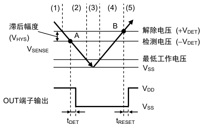
图22 S-19102/19108系列C型的时序图
