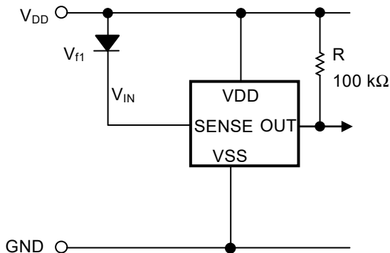
图36 使用二极管后检测电压的改变 (N沟道开路漏极输出产品)
