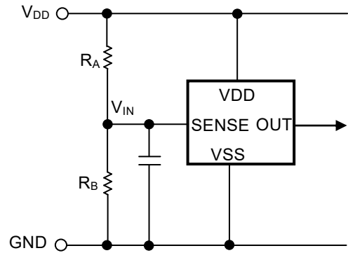
图35 使用分割电阻后检测电压的改变 (CMOS输出产品)
