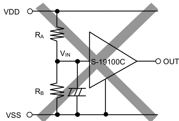
图21 检测电压改变电路不良事例
