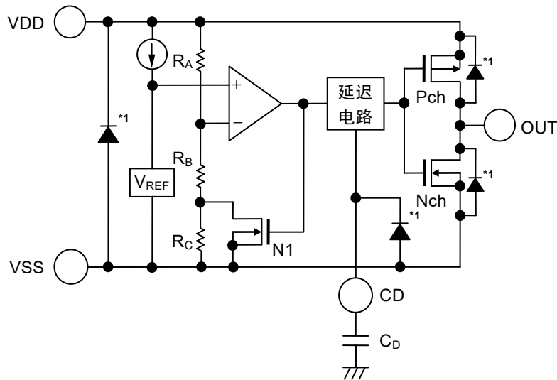
图13 工作说明图1
