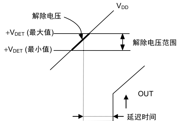
图18 解除电压
