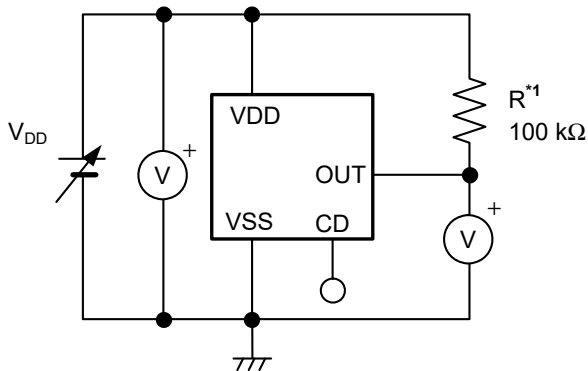
图6 测定电路1
