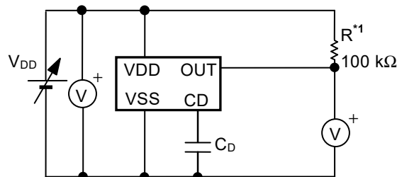
图19 检测电压、解除电压的测定电路
