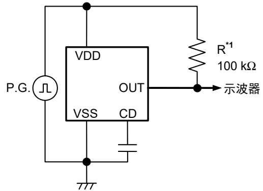
图9 测定电路4
