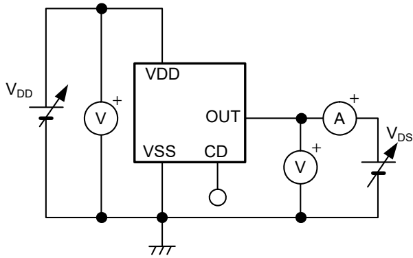
图8 测定电路3
