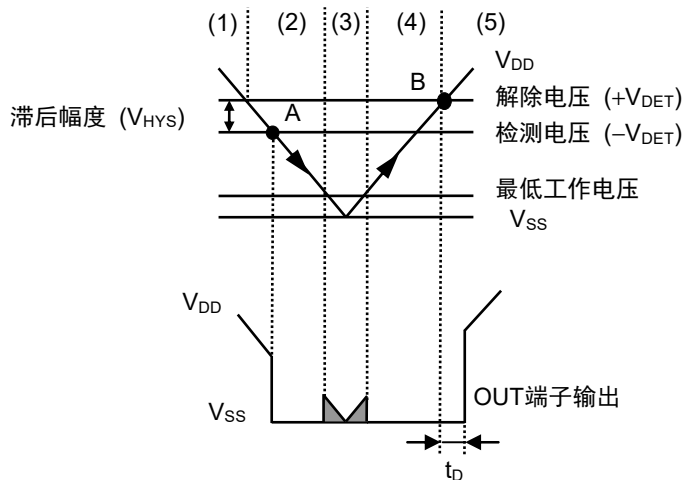
图14 工作说明图2
