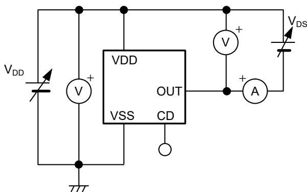
图10 测定电路5
