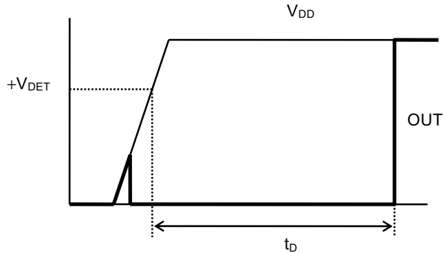
图20 延迟时间
