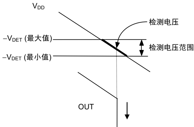
图17 检测电压
