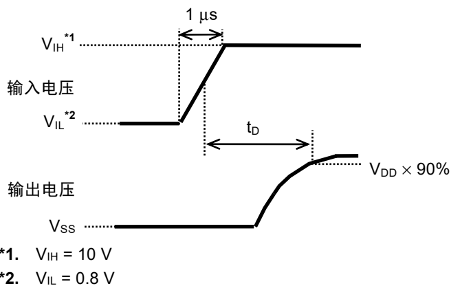
图24 延迟时间的测定条件
