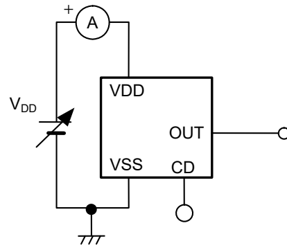
图7 测定电路2
