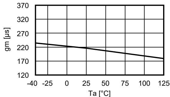
2.13 跨导误差放大电路 ( g_m ) – 温度 ( T_a )
