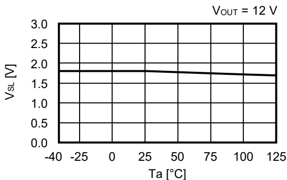
2.12 低电位输入电压 ( V_{SL} ) – 温度 ( T_a )
