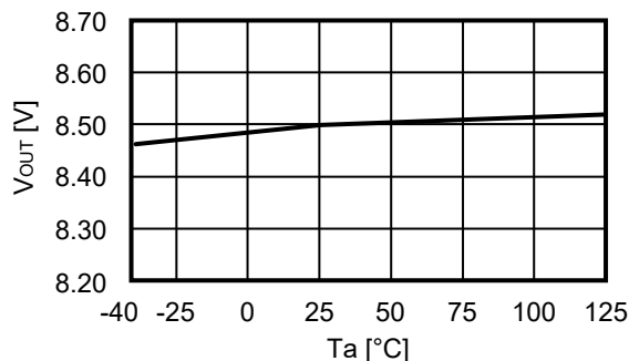
2.14.2 S-19999系列B / D型
