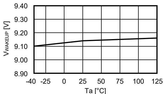
2.15.2 S-19999系列B / D型
