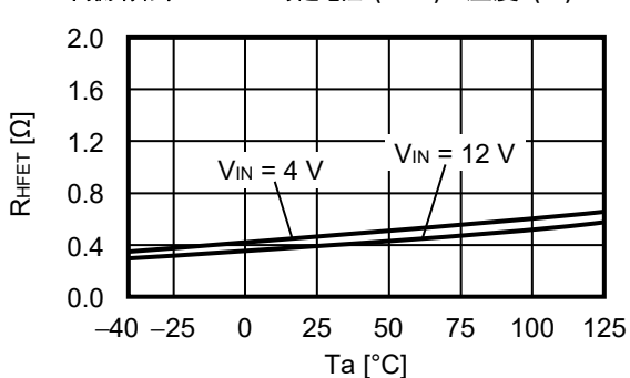
2.9 高侧端功率MOS FET导通电阻 ( R_{HFET} ) – 温度 ( T_a )
