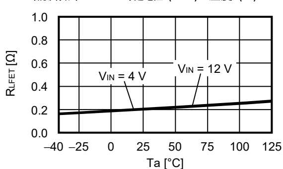
2.10 低侧端功率MOS FET导通电阻 ( R_{LFET} ) – 温度 ( T_a )
